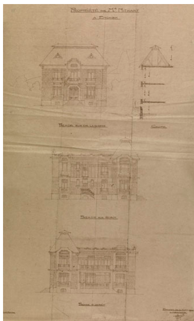
Elévation de trois façades, sur les rues de la Barre, Robin et sur le jardin et coupe par l'architecte Moreels, 1927 (AM Enghien-les-Bains, 1T15)
