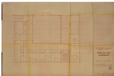
Plan du 2e étage. 1948 Tirage. (AM Mantes-la-Jolie 1M 7) IVR11_20157800410NUC4A
