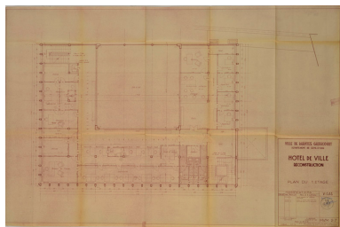
Plan du 1er étage. 1948 Tirage. (AM Mantes-la-Jolie 1M 7) IVR11_20157800409NUC4A
