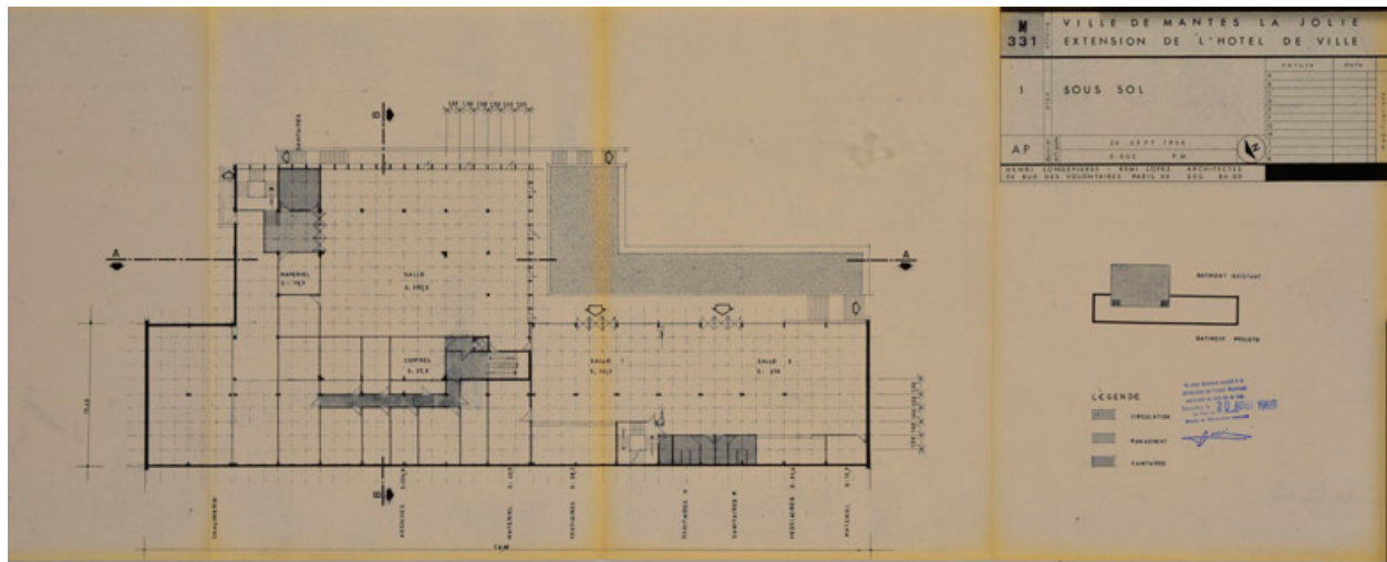
Plan du sous-sol de l'extension. 1968 (AM Mantes-la-Jolie 1M 7)
