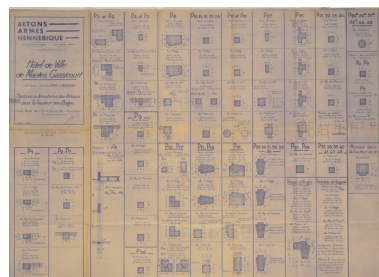
Section des poteaux de l'étage par Les bétons armés Hennebique. 1949. (AM Mantes-la-Jolie 1M 7) IVR11_20157800418NUC4A
