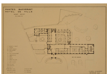
Avant projet (non réalisé). Plan du rez-de-chaussée. Tirage. (AM Mantes-la-Jolie 1M 7) IVR11_20157800401NUC4A
