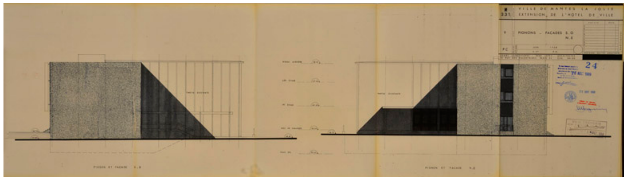
Pignons des façades sud-ouest et nord-est de l'extension. 1968 (AM Mantes-la-Jolie 1M 7)
