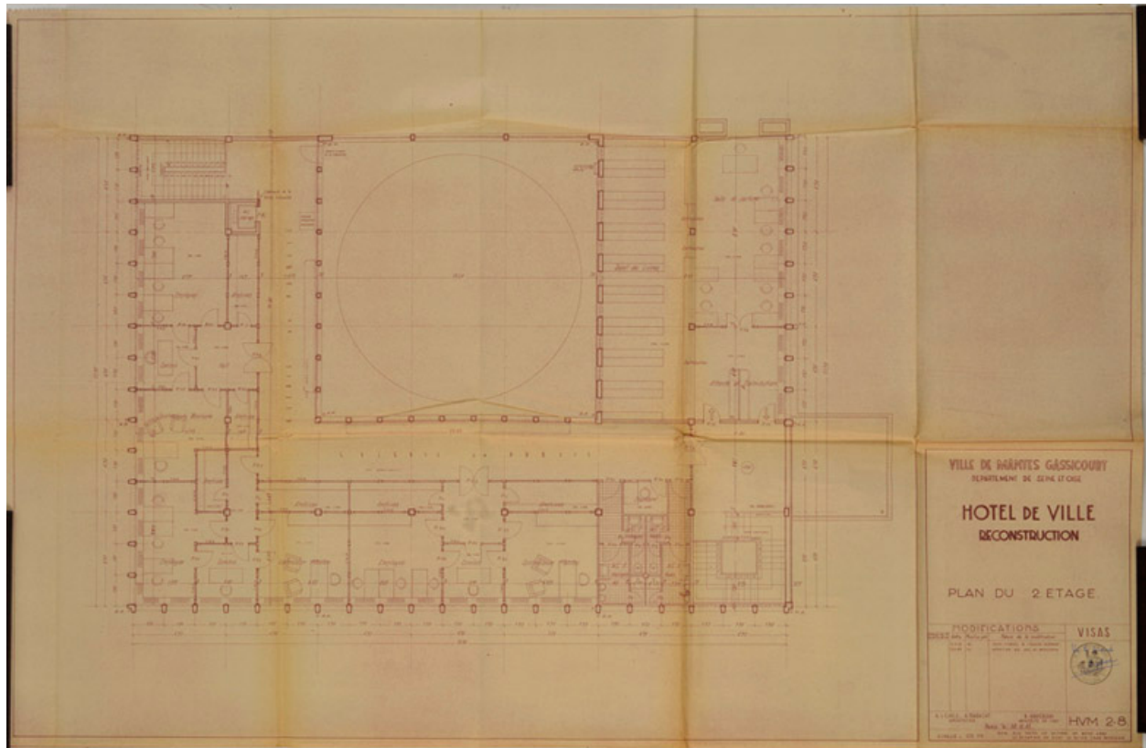
Plan du 2e étage. 1948 Tirage. (AM Mantes-la-Jolie 1M 7)
