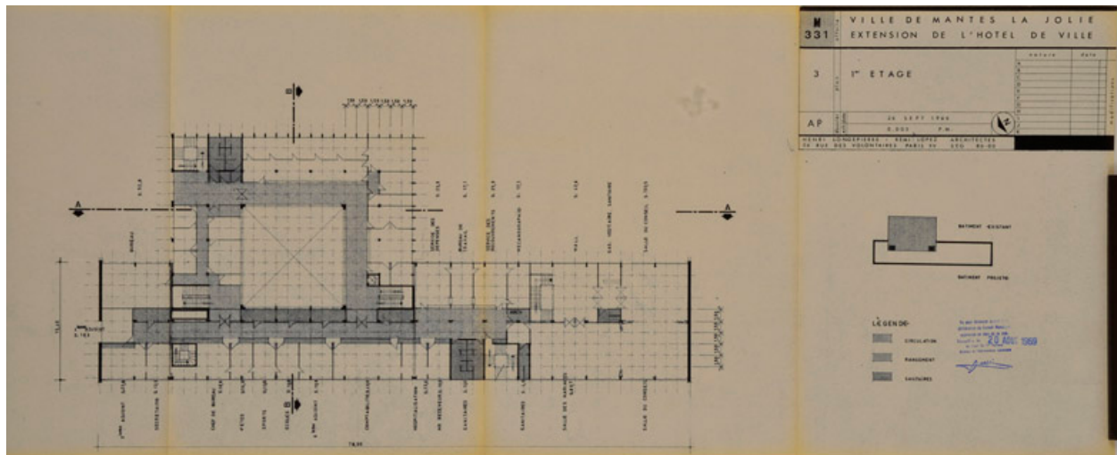
Plan du 1er étage de l'extension. 1968 (AM Mantes-la-Jolie 1M 7)
