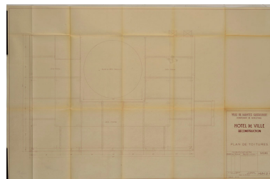
Plan des toitures. 1948 Tirage. (AM Mantes-la-Jolie 1M 7) IVR11_20157800411NUC4A
