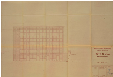
Élévation de la façade sud-ouest. 1948 Tirage. (AM Mantes-la-Jolie 1M 7) IVR11_20157800413NUC4A
