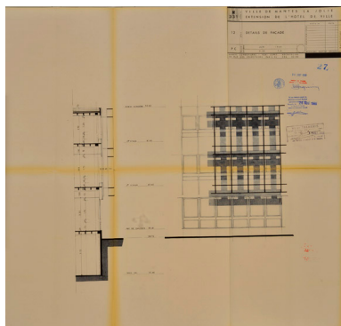
Détails de façade de l'extension. 1968 (AM Mantes-la-Jolie 1M 7) IVR11_20157800427NUC4A
