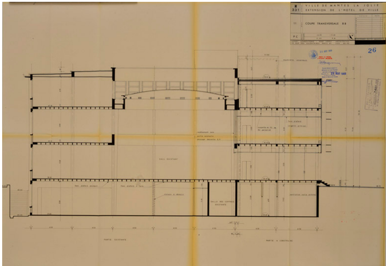
Coupe transversale de l'extension. 1968 (AM Mantes-la-Jolie 1M 7)
