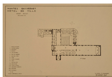
Avant projet (non réalisé). Plan du premier étage. Tirage. (AM Mantes-la-Jolie 1M 7) IVR11_20157800402NUC4A
