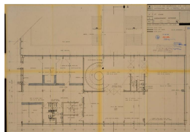
Plan de l'extension. Aménagement intérieur du 1er étage. 1968. (AM Mantes-la-Jolie, 1M 15) IVR11_20157800434NUC4A
