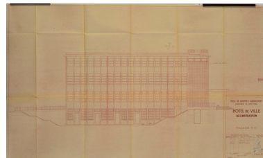
Élévation de la façade sud-est. 1948 Tirage. (AM Mantes-la-Jolie 1M 7) IVR11_20157800414NUC4A
