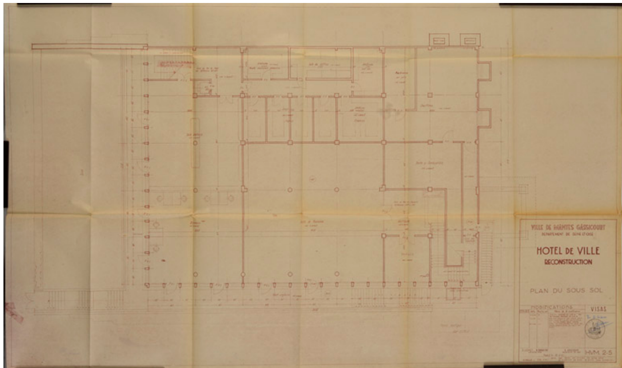
Plan du sous-sol. 1948 Tirage. (AM Mantes-la-Jolie 1M 7)
