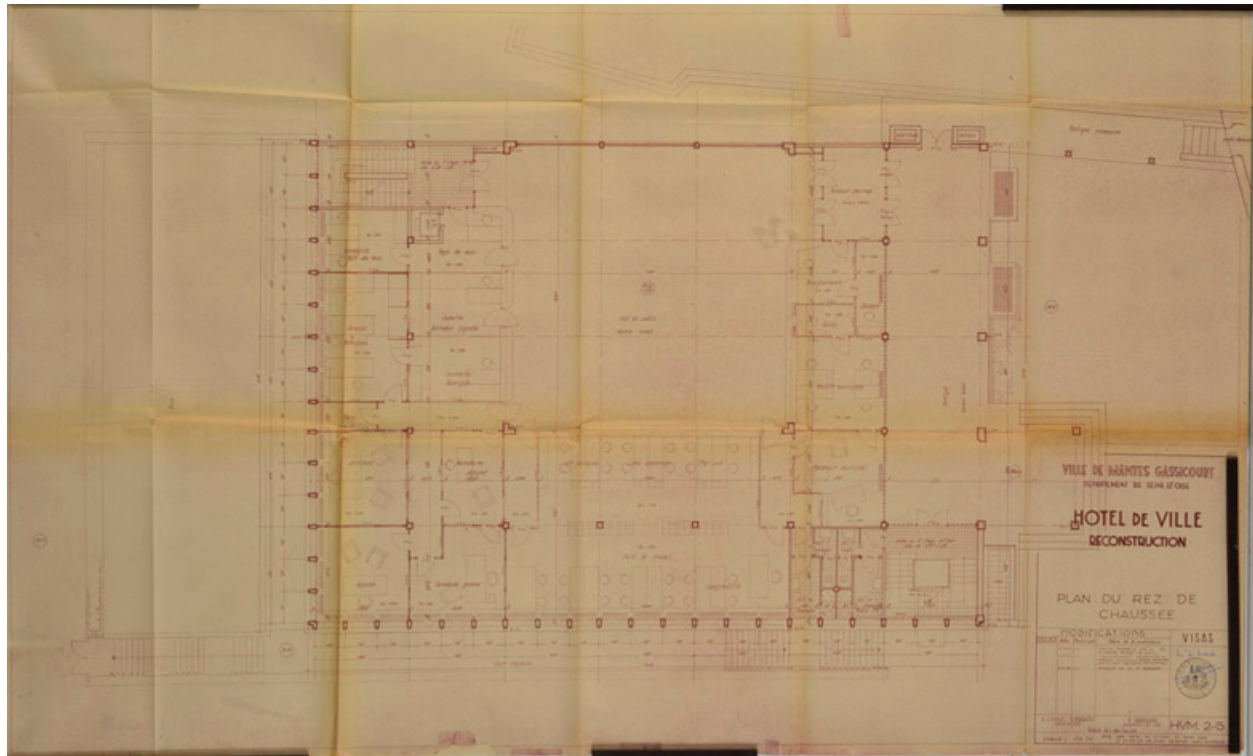
Plan du rez-de-chaussée. 1948 Tirage. (AM Mantes-la-Jolie 1M 7)
