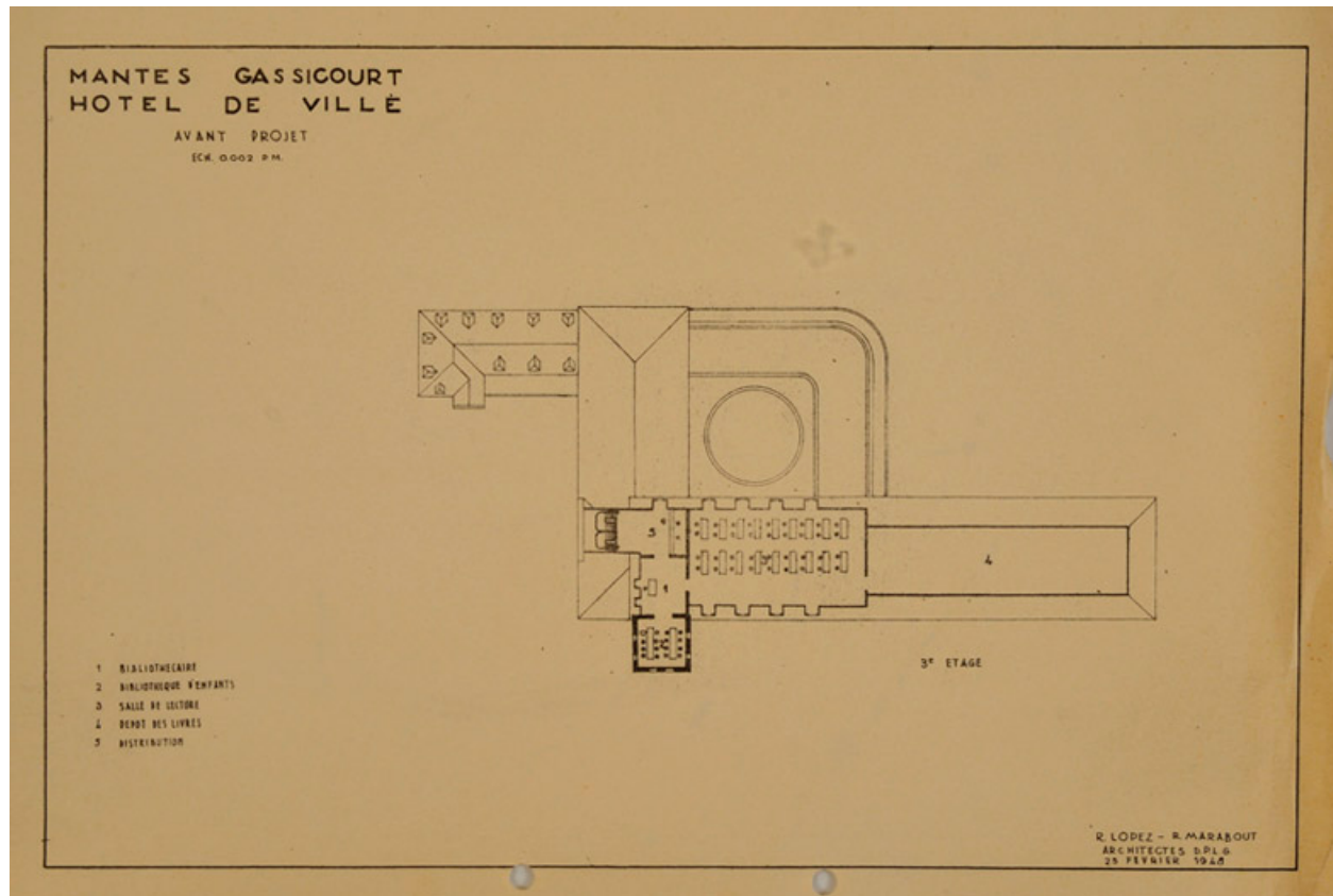
Avant projet (non réalisé). Plan du 3e étage. Tirage. (AM Mantes-la-Jolie 1M 7)
