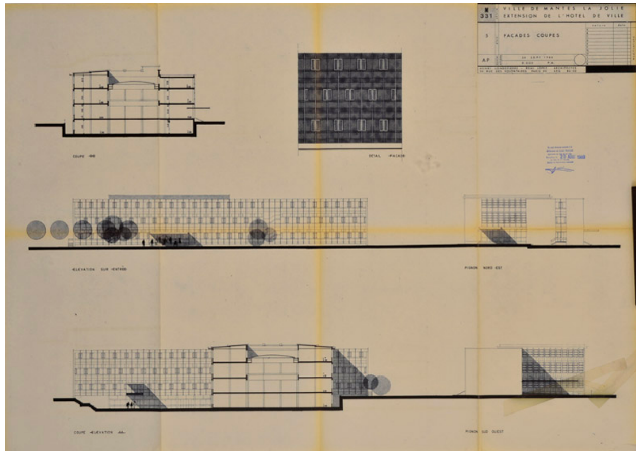
Façades et coupes de l'extension. 1968 (AM Mantes-la-Jolie 1M 7)
