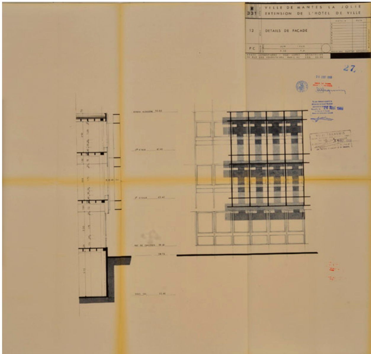
Détails de façade de l'extension. 1968 (AM Mantes-la-Jolie 1M 7)
