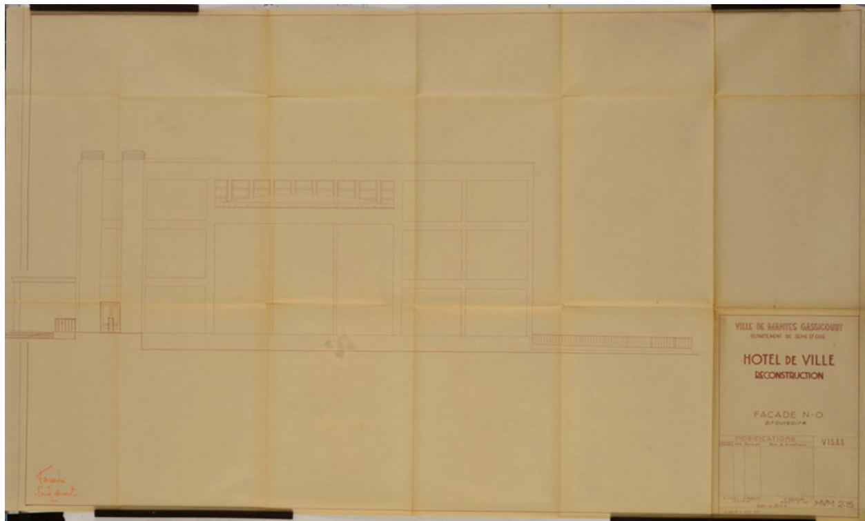
Élévation de la façade nord-ouest. 1948 Tirage. (AM Mantes-la-Jolie 1M 7)
