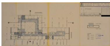
Plan du 2e étage de l'extension. 1968 (AM Mantes-la-Jolie 1M 7) IVR11_20157800424NUC4A
