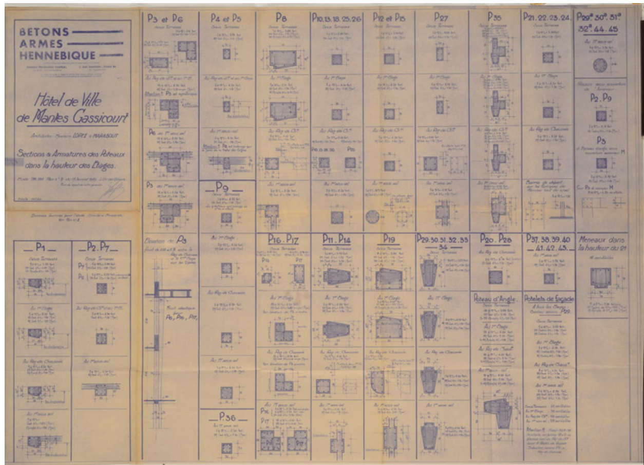
Section des poteaux de l'étage par Les bétons armés Hennebique. 1949. (AM Mantes-la-Jolie 1M 7)
