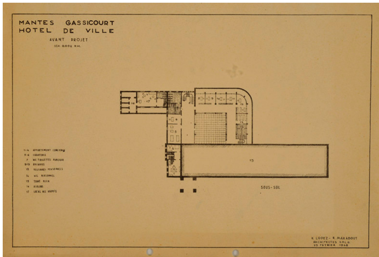
Avant projet (non réalisé). Plan du sous-sol. Tirage. (AM Mantes-la-Jolie 1M 7)
