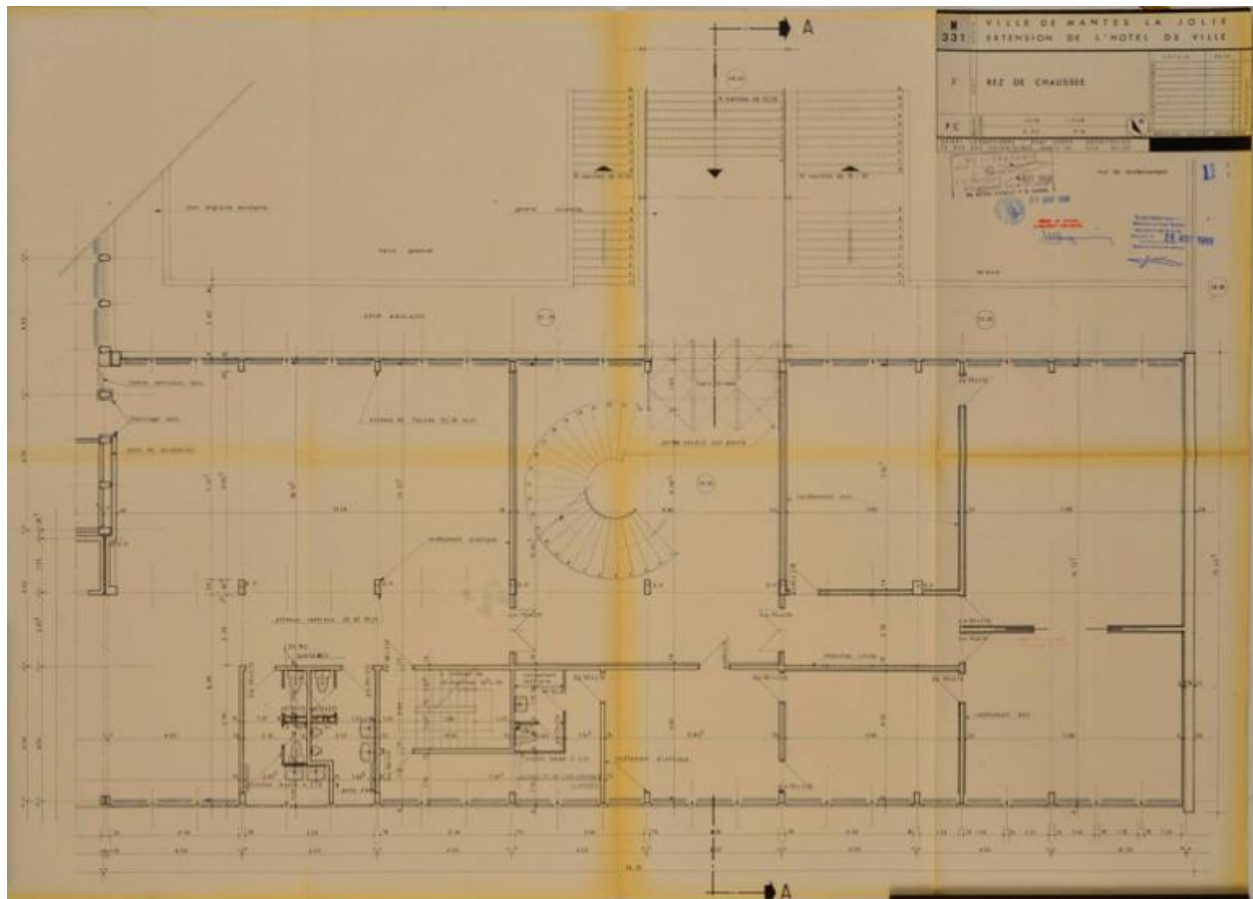
Plan de l'extension. Rez-de-chaussée. 1968. (AM Mantes-la-Jolie, 1M 15)
