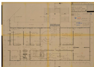
Plan de l'extension. Aménagement intérieur du rez-de-chaussée. 1968. (AM Mantes-la-Jolie, 1M 15) IVR11_20157800435NUC4A
