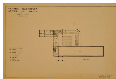
Avant projet (non réalisé). Plan du sous-sol. Tirage. (AM Mantes-la-Jolie 1M 7) IVR11_20157800405NUC4A
