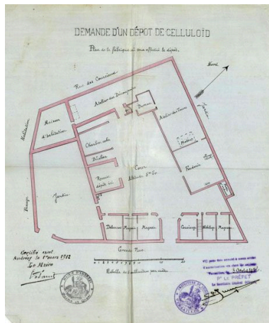
Plan de distribution à l'époque de l'usine de jouets en 1912. (AD Yvelines, 7 M 105). Repro. Archives départementales des Yvelines IVR11_20087800658NUC2A
