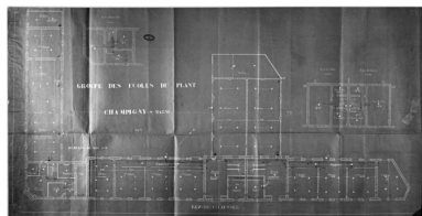
Plan du rez-de-chaussée, 1923. (Archives de Paris. DO 3 50) Phot. Philippe Rivière IVR11_19869400508P
