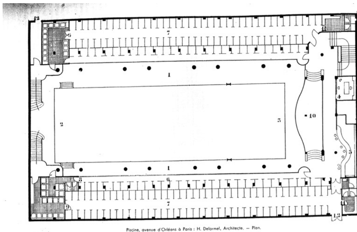
Plan général de la piscine. La Construction moderne, 10 février 1935
