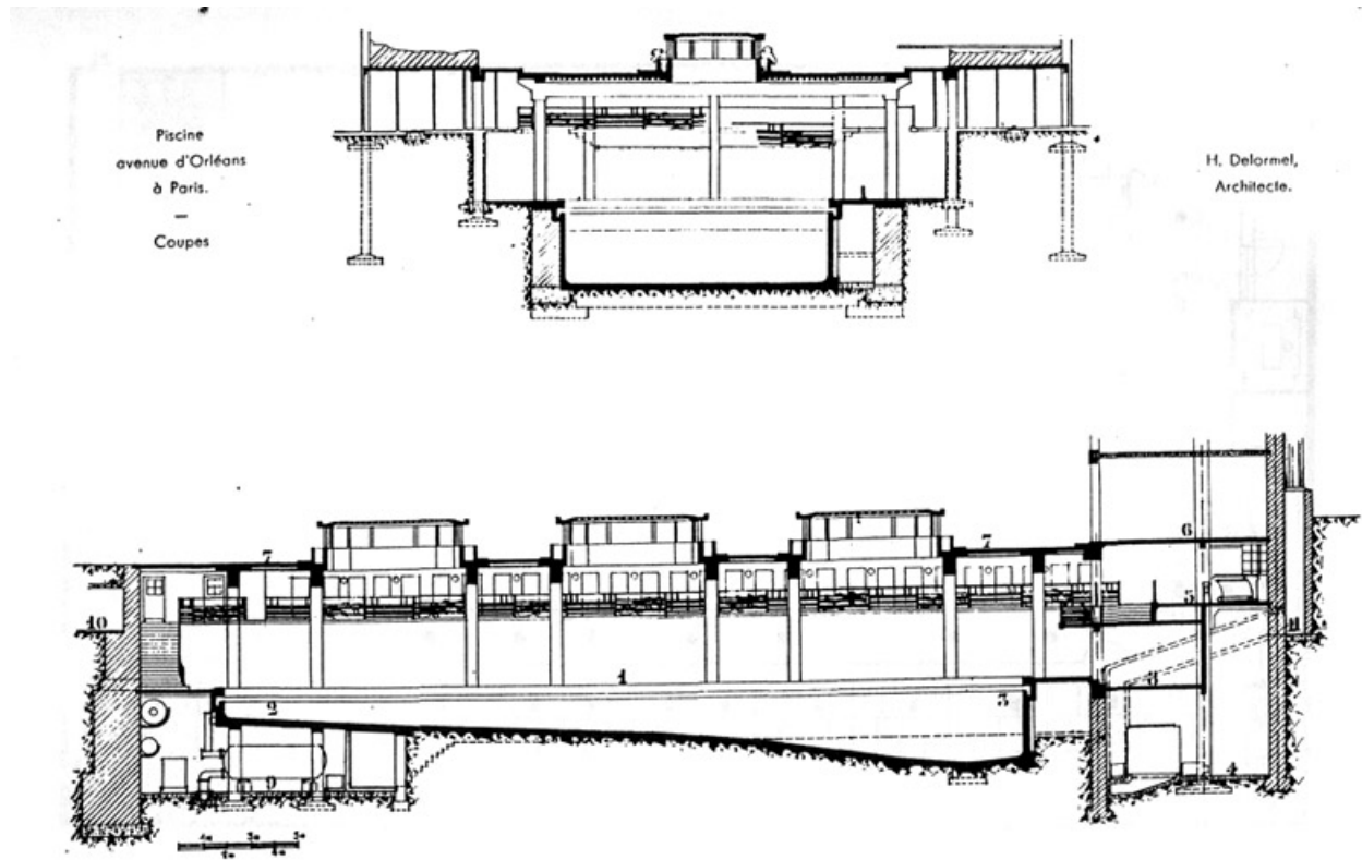
Coupes longitudinale et transversale de la piscine. La Construction moderne, 10 février 1935
