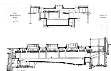
Coupes longitudinale et transversale de la piscine. La Construction moderne, 10 février 1935 IVR11_20157500309NUC4A
