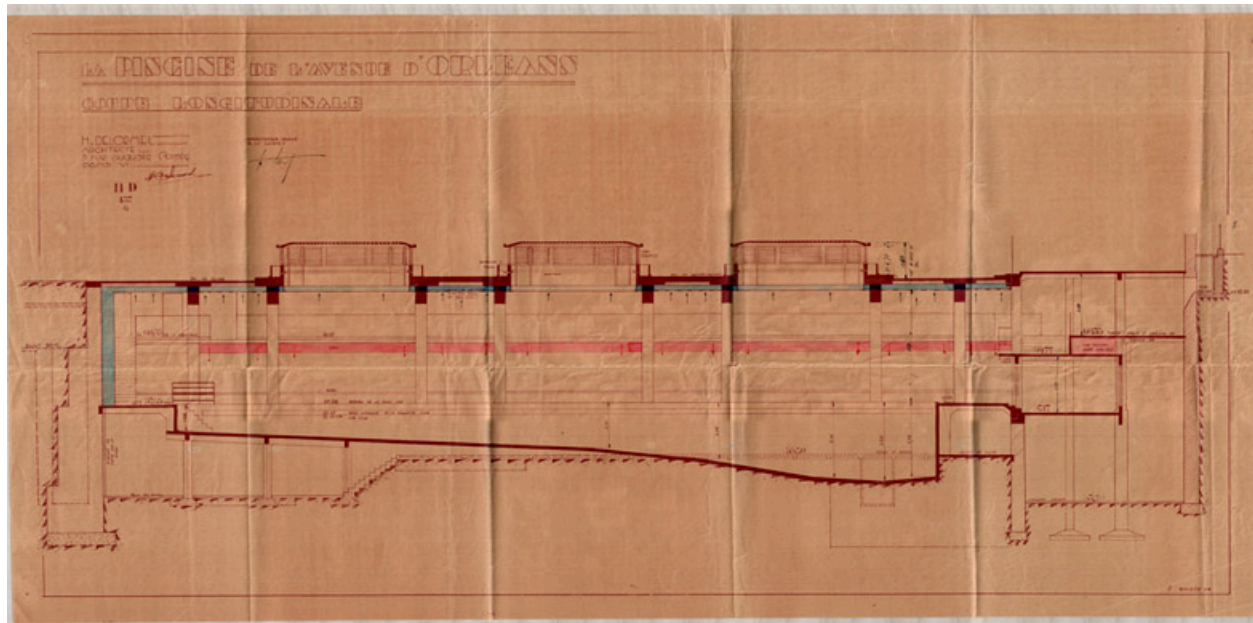
Coupe longitudinale de la piscine dressée par H.Delormel, 1934. (Archives de Paris. VO 11 2486)
