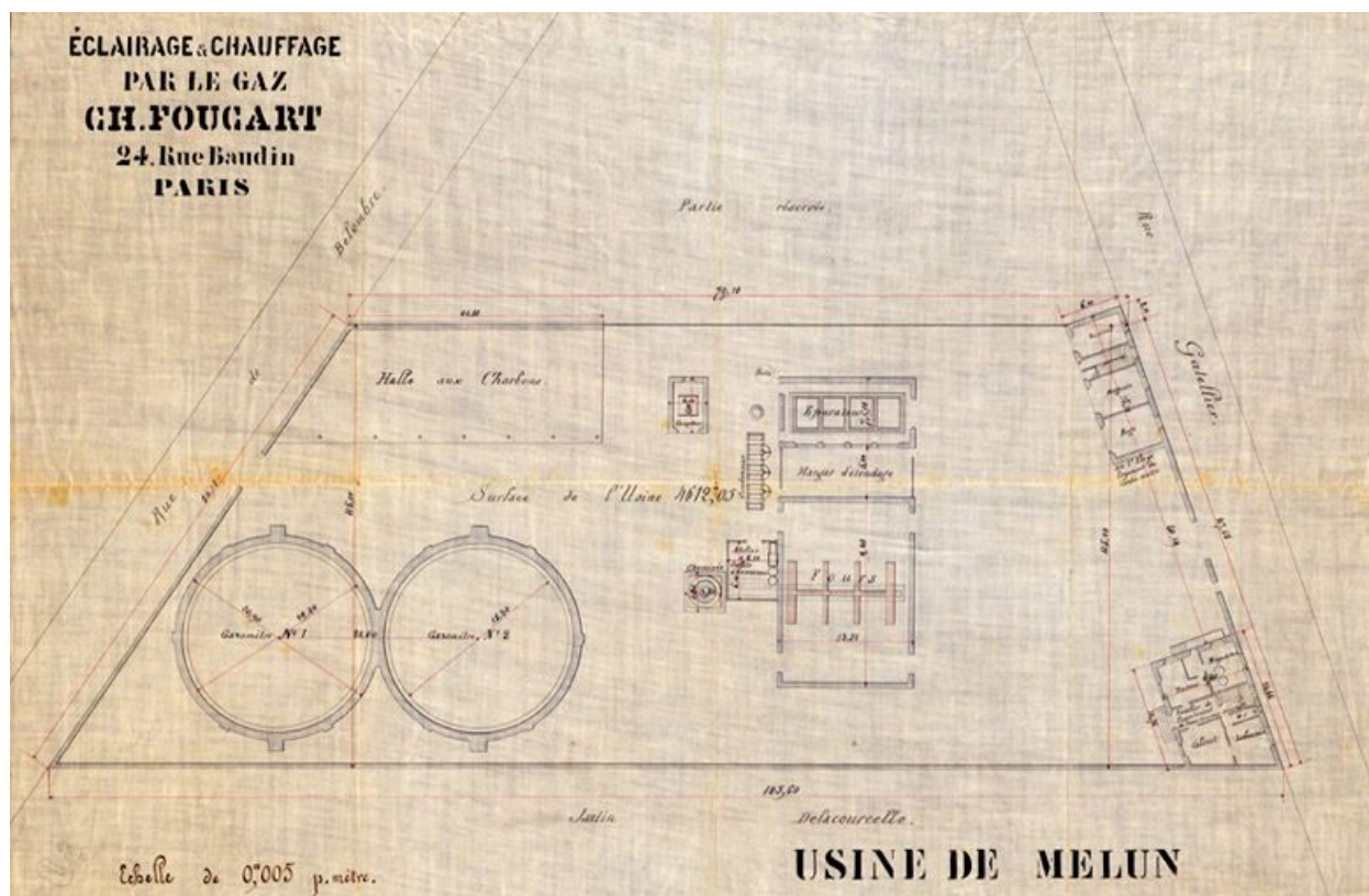
Plan de l'usine à gaz à l'angle de la rue de Belombre et de la rue Gatellier (aujourd'hui disparue) : "Eclairage et chauffage par le gaz Ch. Foucart (24 rue Baudin. Paris). Usine de Melun." 19e siècle. (AM Melun. 1 Fi 1461)
