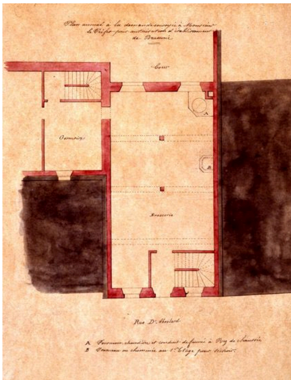
Projet d'installation de la brasserie par Jacob. Calque aquarellé, 1851. (AD Seine-et-Marne. 5 Mp 295)
