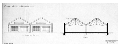
Usine ""Messieurs Blériot et Devoisselle (imprimerie, cartons) : façade, coupe. Papier, tirage d'architecte, 1937. (AM Melun. 1 Fi 1549) Phot. Archives municipales de Melun (reproduction), Autr. G.(architecte) Cabaret IVR11_20047700381NUC
