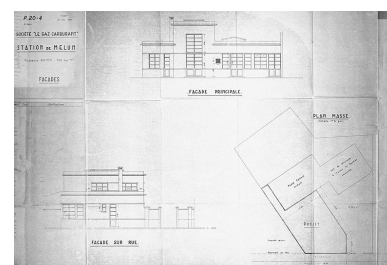
Station de Melun : façades (éch. 1/50e) et plan masse (éch. 0,01 p.m.), 21 mai 1941. ""Papier, tirage d'architecte, 1941. (AM Melun. 1 Fi 2300) Phot. Archives municipales de Melun (reproduction), Autr. R. Blanc IVR11_20047700541NUC
