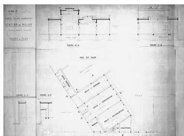
Station de Melun : coupes et plan de l'aile projetée, échelle 1/50e, 16 mai 1941. "" .Papier, tirage d'architecte, 1941. (AM Melun. 1 Fi 2302) Phot. Archives municipales de Melun (reproduction), Autr. R. Blanc IVR11_20047700543NUC
