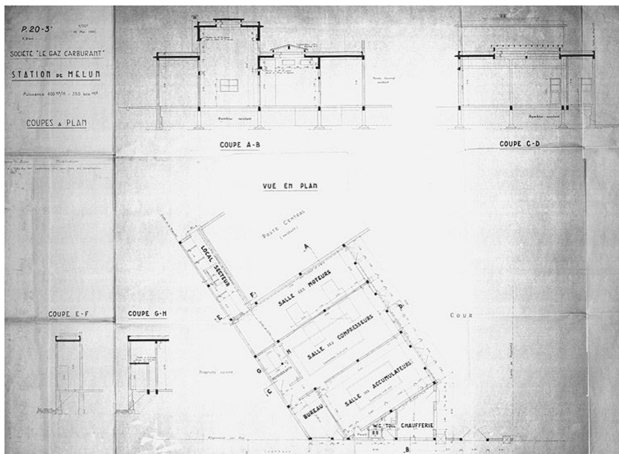
Station de Melun : coupes et plan de l'aile projetée, échelle 1/50e, 16 mai 1941". Papier, tirage d'architecte, 1941. (AM Melun. 1 Fi 2302)
