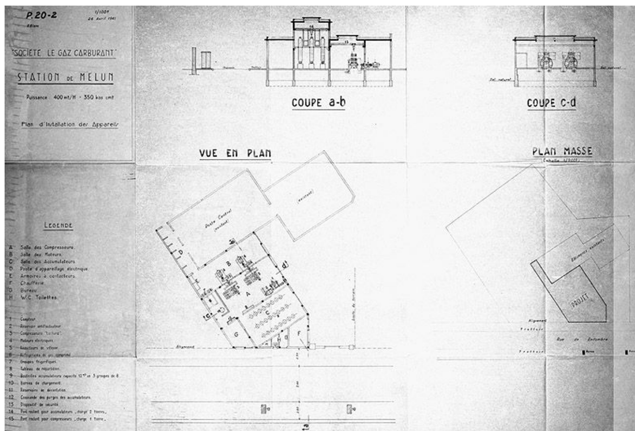
Station de Melun : plan d'installation des appareils, échelle 1/100e, 26 avril 1941. "" .Papier, tirage d'architecte, 1941. (AM Melun. 1 Fi 2301)
