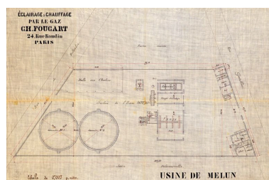
Plan de l'usine à gaz à l'angle de la rue de Belombre et de la rue Gatelliet (aujourd'hui disparue) : ""Eclairage et chauffage par le gaz Ch. Foucart (24 rue Baudin. Paris). Usine de Melun. ""19e siècle. (AM Melun. 1 Fi 1461) Phot. Archives municipales de Melun (reproduction) IVR11_20047700370NUCA
