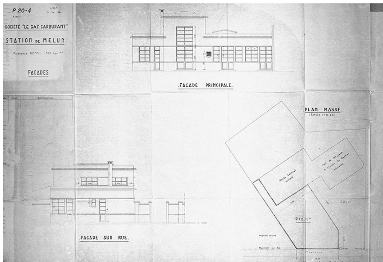
Station de Melun : façades (éch. 1/50e) et plan masse (éch. 0,01 p.m.), 21 mai 1941. ""Papier, tirage d'architecte, 1941. (AM Melun. 1 Fi 2300)
