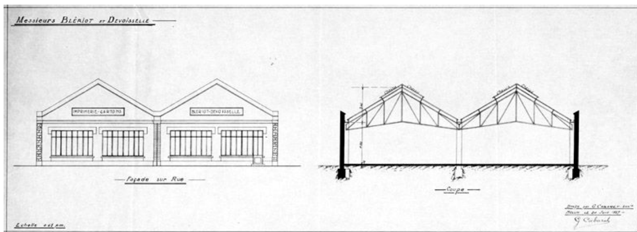
Usine ""Messieurs Blériot et Devoisselle (imprimerie, cartons) : façade, coupe. Papier, tirage d'architecte, 1937. (AM Melun. 1 Fi 1549)
