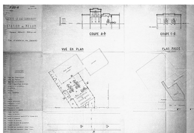
Station de Melun : plan d'installation des appareils, échelle 1/100e, 26 avril 1941. "" .Papier, tirage d'architecte, 1941. (AM Melun. 1 Fi 2301) Phot. Archives municipales de Melun (reproduction), Autr. R. Blanc IVR11_20047700542NUC
