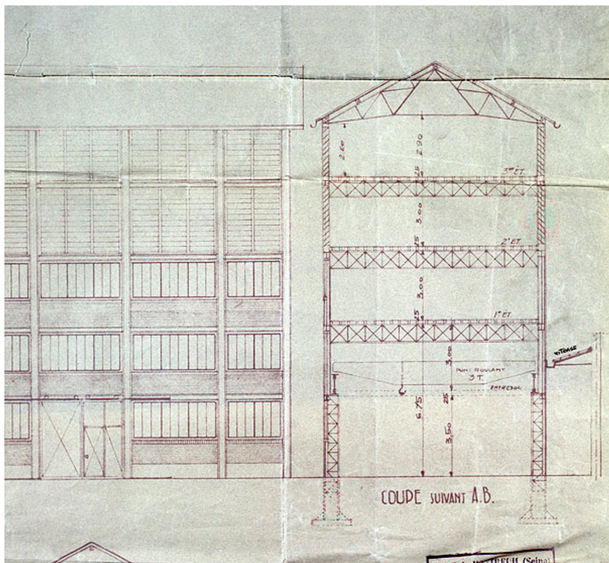
Coupe et profil de la scierie Treuil et Gasq. Plan, 1929. (AM Montreuil)
