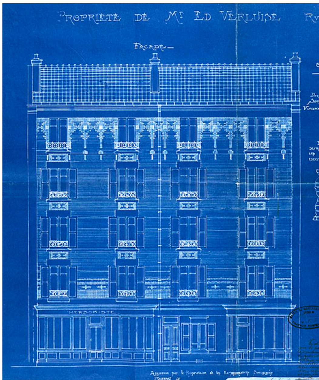
Plan bleu, façade maison Verluise. (AM Montreuil)
