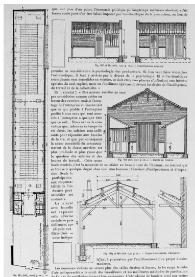
Etablissement industriel (plan, coupes, élévations). Gravure. Tiré de : L'Architecture usuelle, 1923. (BHVP) Autr. E. Lemerre (architecte) IVR11_20029300301X
