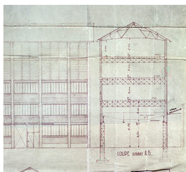
Coupe et profil de la scierie Treuil et Gasq. Plan, 1929. (AM Montreuil) IVR11_20079300036XA
