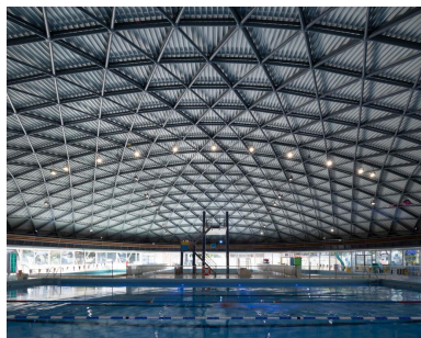
Stade nautique de Drancy. Charpente métallique. Phot. Ayrault Philippe IVR11_20229300863NUC4A
