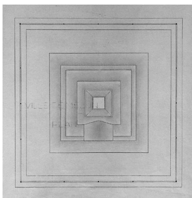
Plan du socle. Encre sur papier, 10 juin 1943. (AM Melun. 1 Fi 77 (verso)) Phot. Philippe Ayrault IVR11_20027700006X
