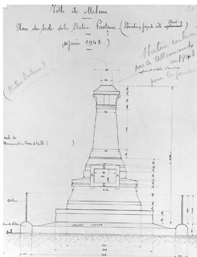
Socle du monument à Pasteur : élévation nord. Encre sur papier, 10 juin 1943. (AM Melun. 1 Fi 77 (recto)) Phot. Philippe Ayrault IVR11_20027700007X
