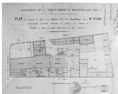
Plan de l'usine en 1897. (AD Seine-Saint-Denis. B NB 111) IVR11_20029300088NUC
