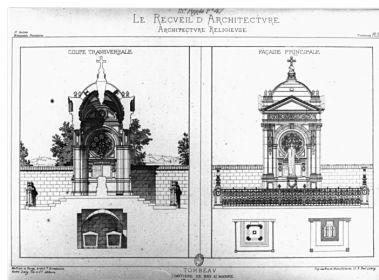
Coupe transversale et élévation antérieure. Tiré de : Recueil d'Architecture, 1887. Autr. M. (architecte) Bir IVR11_19859400494X
