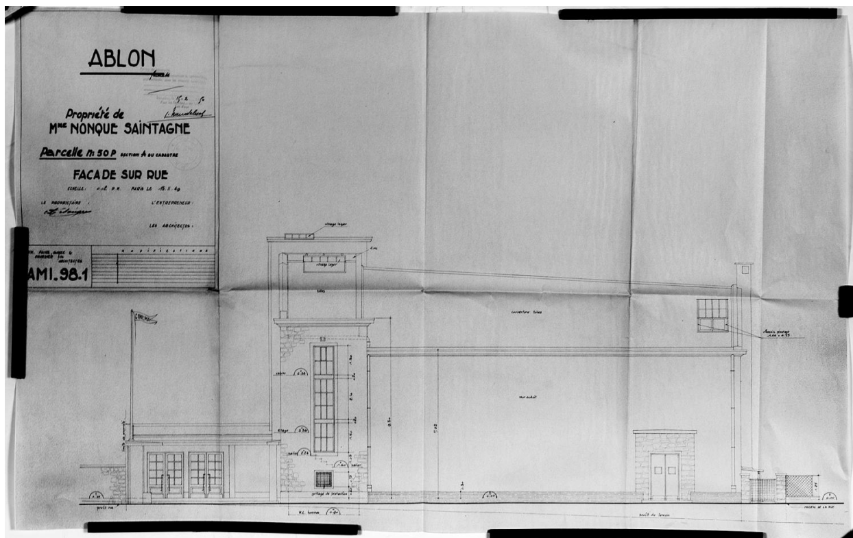
Façade sur rue du cinéma reconstruit pour Mme Nonque à Ablon, à la suite du transfert dans cette commune de ses indemnités de dommages de guerre ; Faine et Gauze, architectes, 15 novembre 1949.
