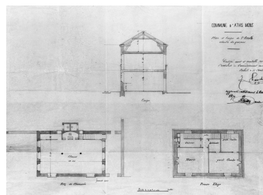
Plan et coupe de la première mairie-école (école de garçons), ruinée par l'occupation allemande de 1870. Elle se situait près du
