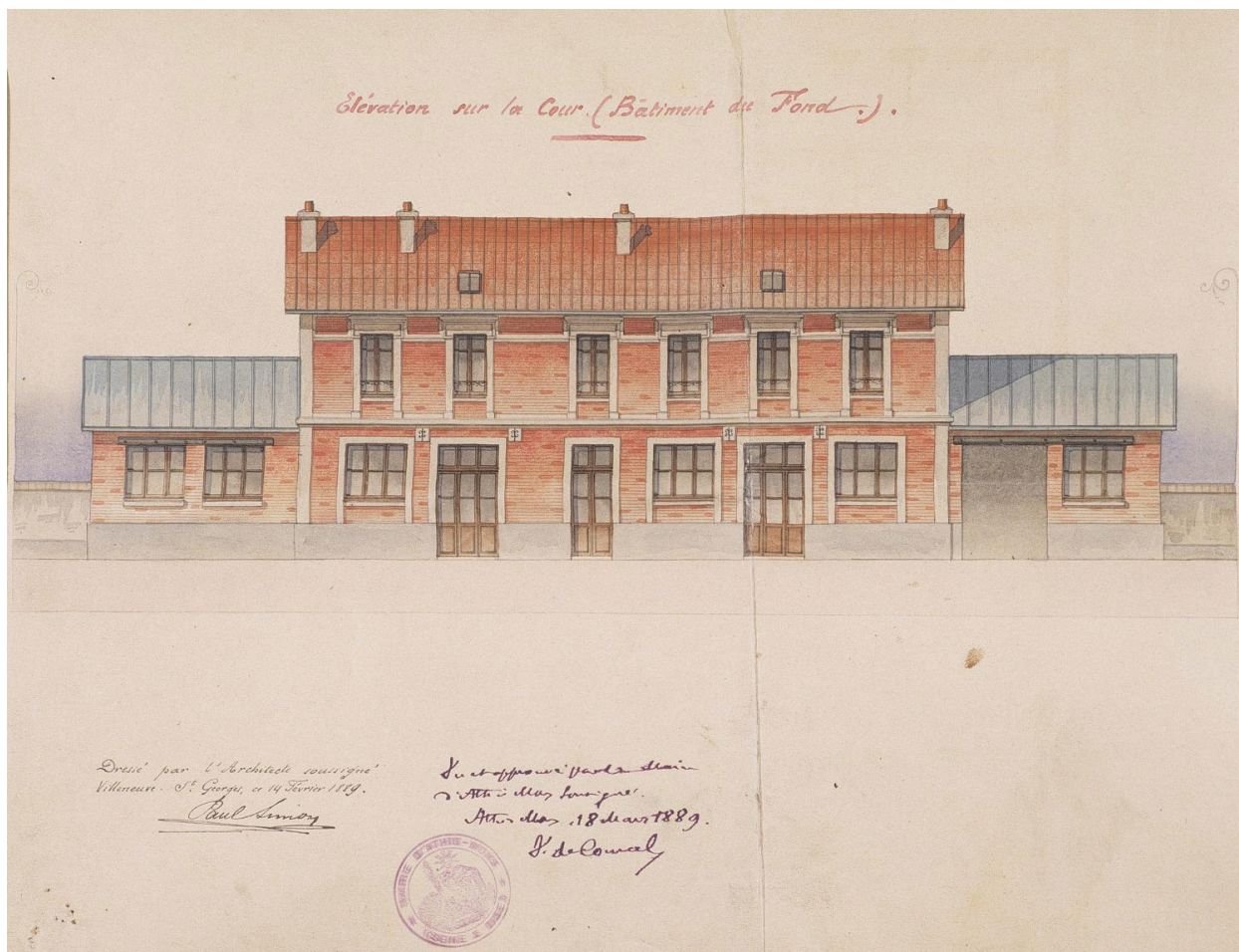
Agrandissement de 1889, détail du plan dressé par Paul Simon : élévation sur la cour du bâtiment du fond. 14 février 1889.
