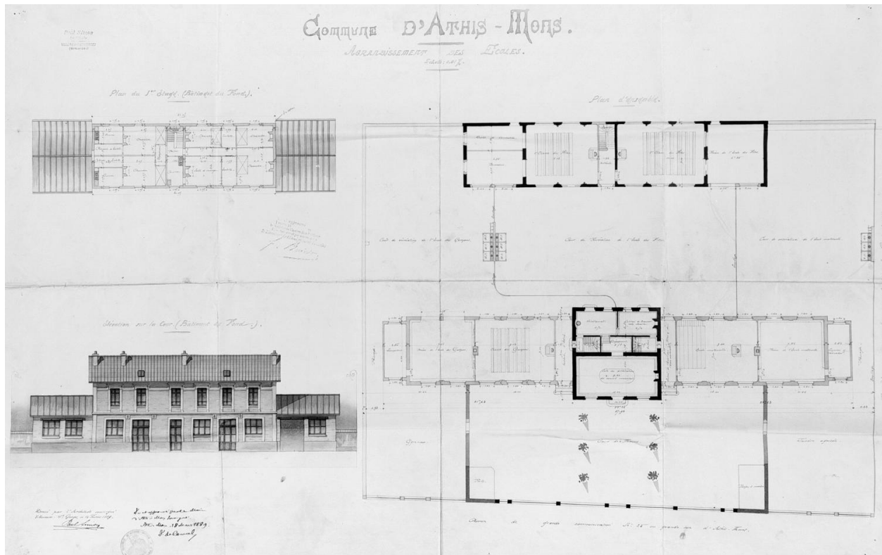
Agrandissement de 1889 : plan d'ensemble, et élévation et 1er étage du bâtiment situé en fond de cour, dressés par l'architecte Paul Simon, 14 février 1889.
