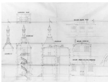
Projet de l'architecte Eugène Tuane : coupes et façades des écoles, 20 juin 1876. IVR11_20029101759X
