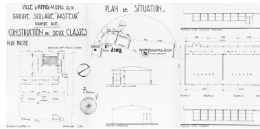
Construction de deux classes en préfabriqué, à l'arrière des bâtiments, entre les ateliers de menuiserie et de serrurerie : plan masse, coupe et élévations ; architectes Thivier et Poggi, septembre 1953. IVR11_20029100713X
