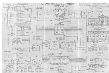
Plan d'ensemble, plans du rez-de-chaussée et du 1er étage des deux corps de bâtiment, élévations et coupes diverses ; octobre 1948. IVR11_20029100673X
