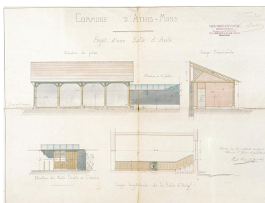
Projet d'une salle d'asile à construire dans l'ancienne école de filles : coupes et élévation ; Simon et Ducastel, architectes, 22 juillet 1882. IVR11_20029101775XA
