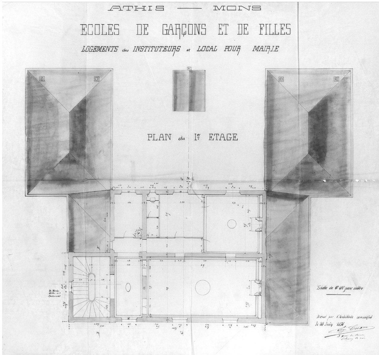
Projet de l'architecte Tuane : plan du 1er étage, 20 juin 1876.
