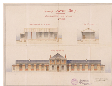
Agrandissement du bâtiment par l'architecte Paul Simon en 1889 : élévation principale et coupes longitudinale et transversale sur un groupe ; 14 février 1889. IVR11_20029100701XA
