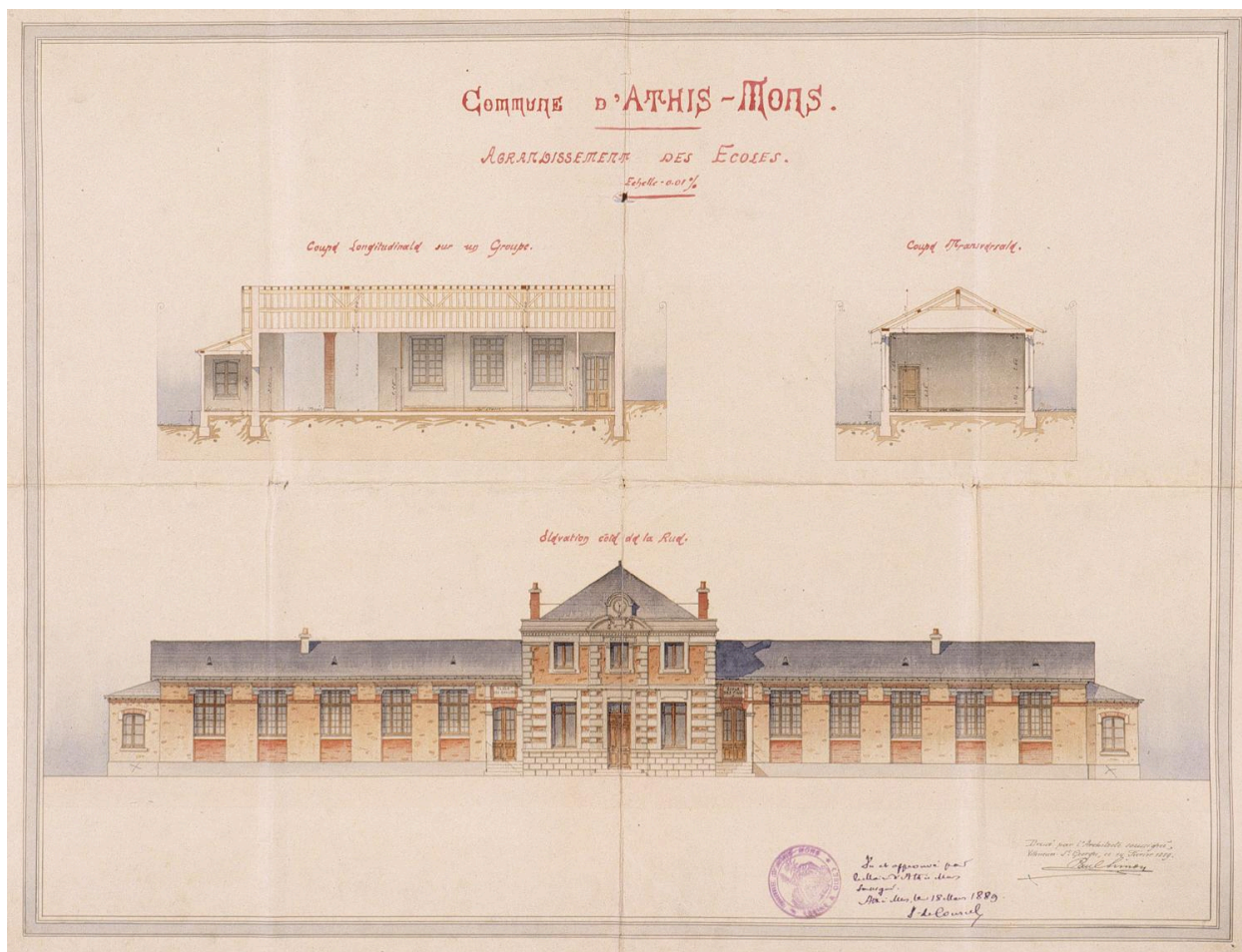
Agrandissement du bâtiment par l'architecte Paul Simon en 1889 : élévation principale et coupes longitudinale et transversale sur un groupe ; 14 février 1889.
