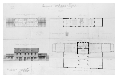
Agrandissement de 1889 : plan d'ensemble, et élévation et 1er étage du bâtiment situé en fond de cour, dressés par l'architecte Paul Simon, 14 février 1889. IVR11_20029100696X
