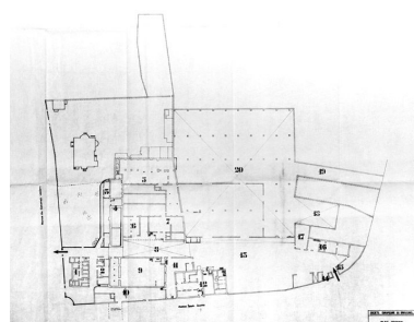
Plan d'ensemble, en 1979 (échelle : 1/400). Phot. Philippe Ayrault IVR11_20037700419X
