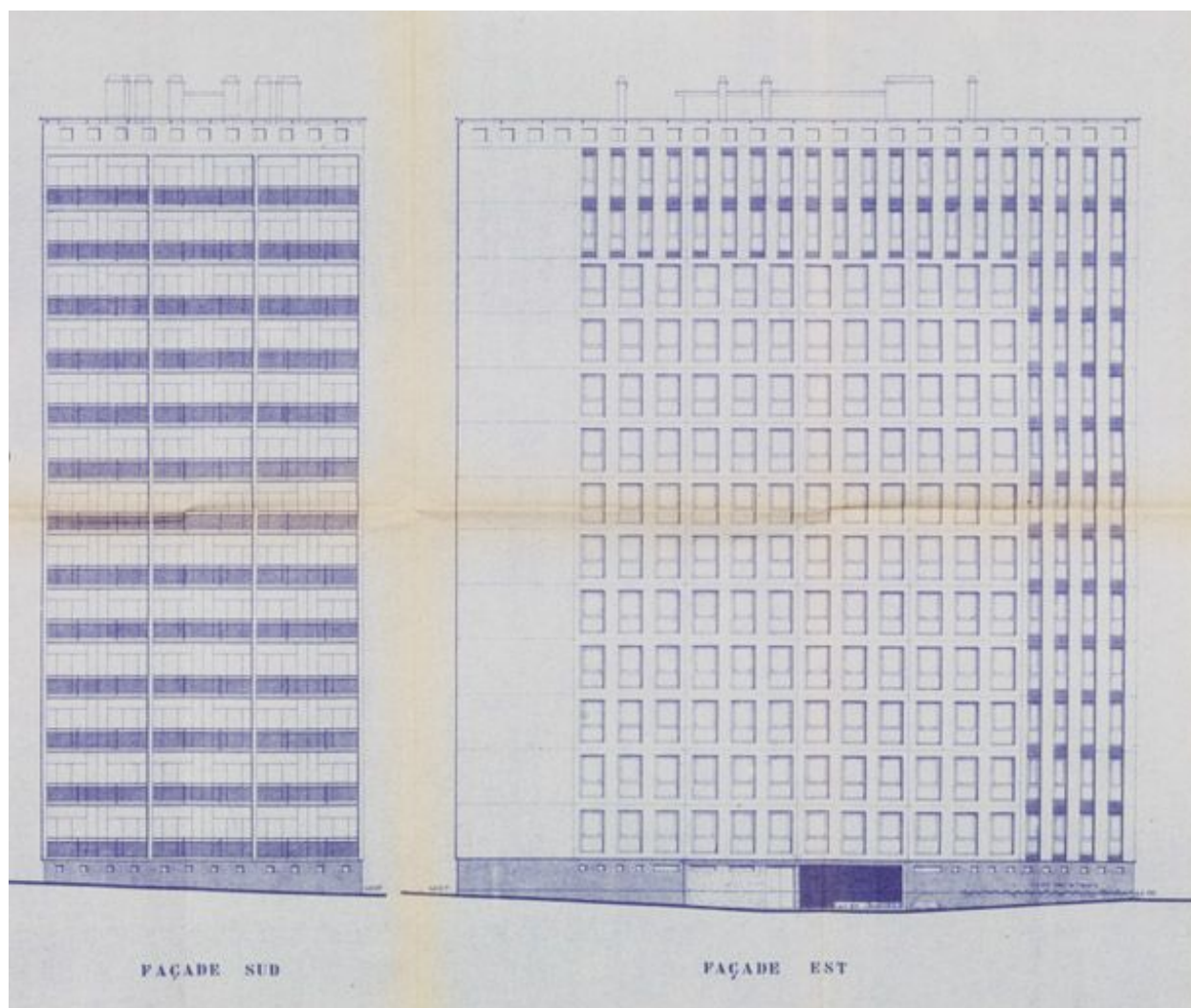
Façades est et sud d'un bâtiment R + 13. (AD Essonne, 1502 W 1277-1278 )
