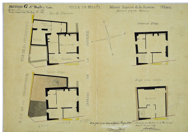
4 plans de la maison Mareau, impasse de la Juiverie, 1885. Papier aquarellé. (AD Seine-et-Marne. 4 Op 284/14) Phot. Yvan Bourhis IVR11_20137700028NUC4A
