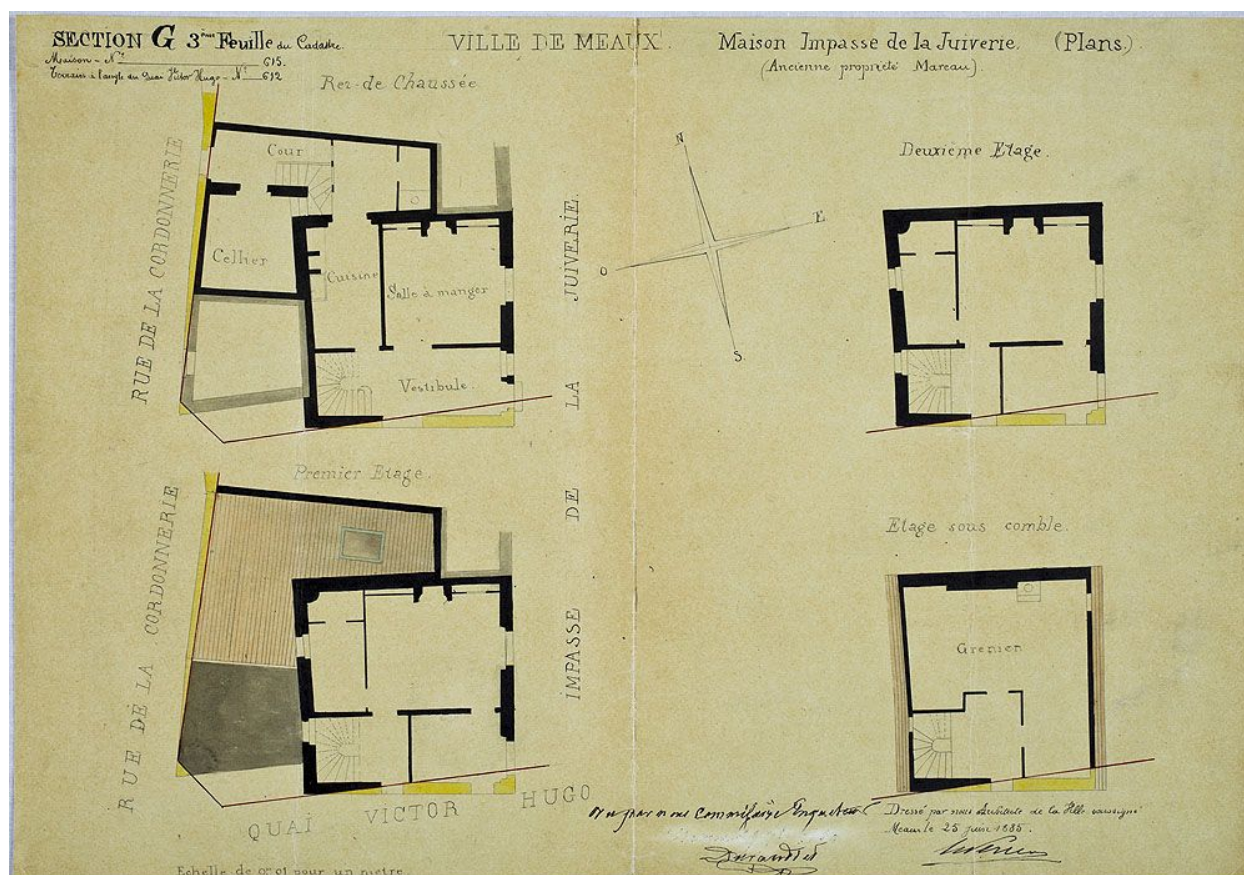
4 plans de la maison Mareau, impasse de la Juiverie, 1885. Papier aquarelléPapier aquarellé. (AD Seine-et-Marne. 4 Op 284/14)
