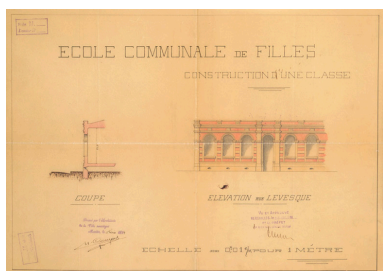
Projet de création d'une classe supplémentaire, élévation. Dessin de l'architecte N.Cauzard.1899 (AM Mantes-la-Jolie, 1 Fi 269) IVR11_20157800519NUC4A
