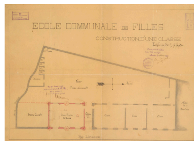
Projet de création d'une classe supplémentaire, plan. Dessin de l'architecte N.Cauzard.1899 (AM Mantes-la-Jolie, 1 Fi 265) IVR11_20157800518NUC4A
