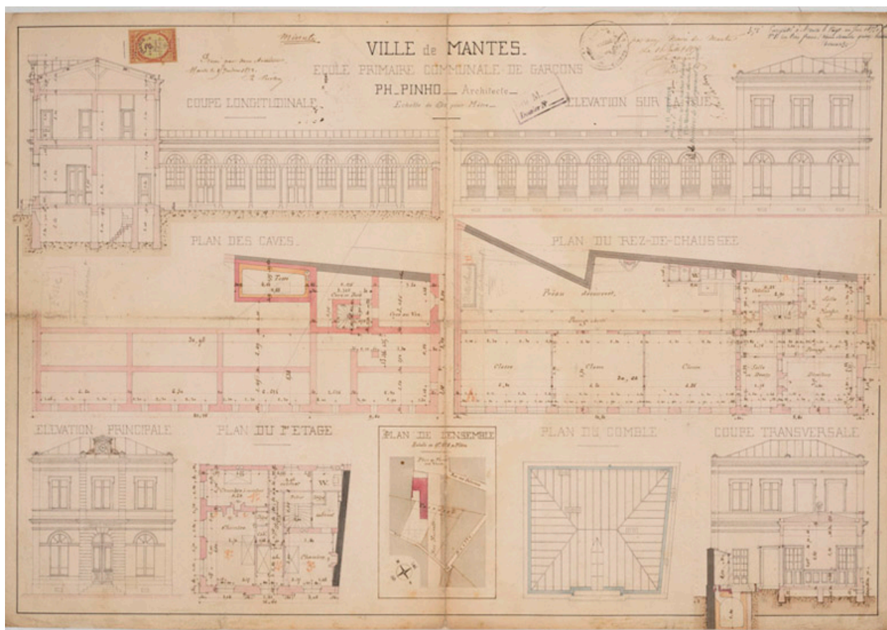
Plans et élévations de l'école. Dessins de Ph. Pinho, architecte, 1873 (AM Mantes-la-Jolie, FI2 64)
