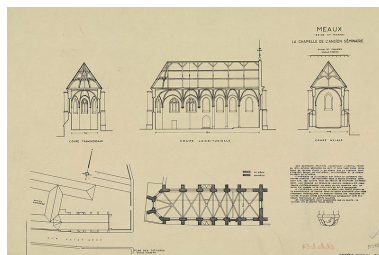
Relevés de P. Barniaud, en 1943 : plan d'ensemble, plan des toitures, coupe axiale, coupes longitudinale et transversale. (Médiathèque de l'architecture et du patrimoine. 0082/077/2019, document n°81975.) Phot. Réunion des musées nationaux, Autr. P. (architecte) Barniaud IVR11_20127701003NUC2A
