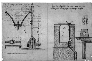
Coupe de l'aqueduc de Buc. IVR11_19957800001P
