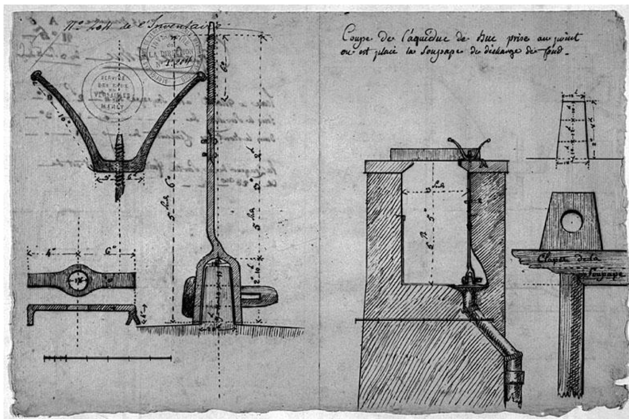
Coupe de l'aqueduc de Buc.
