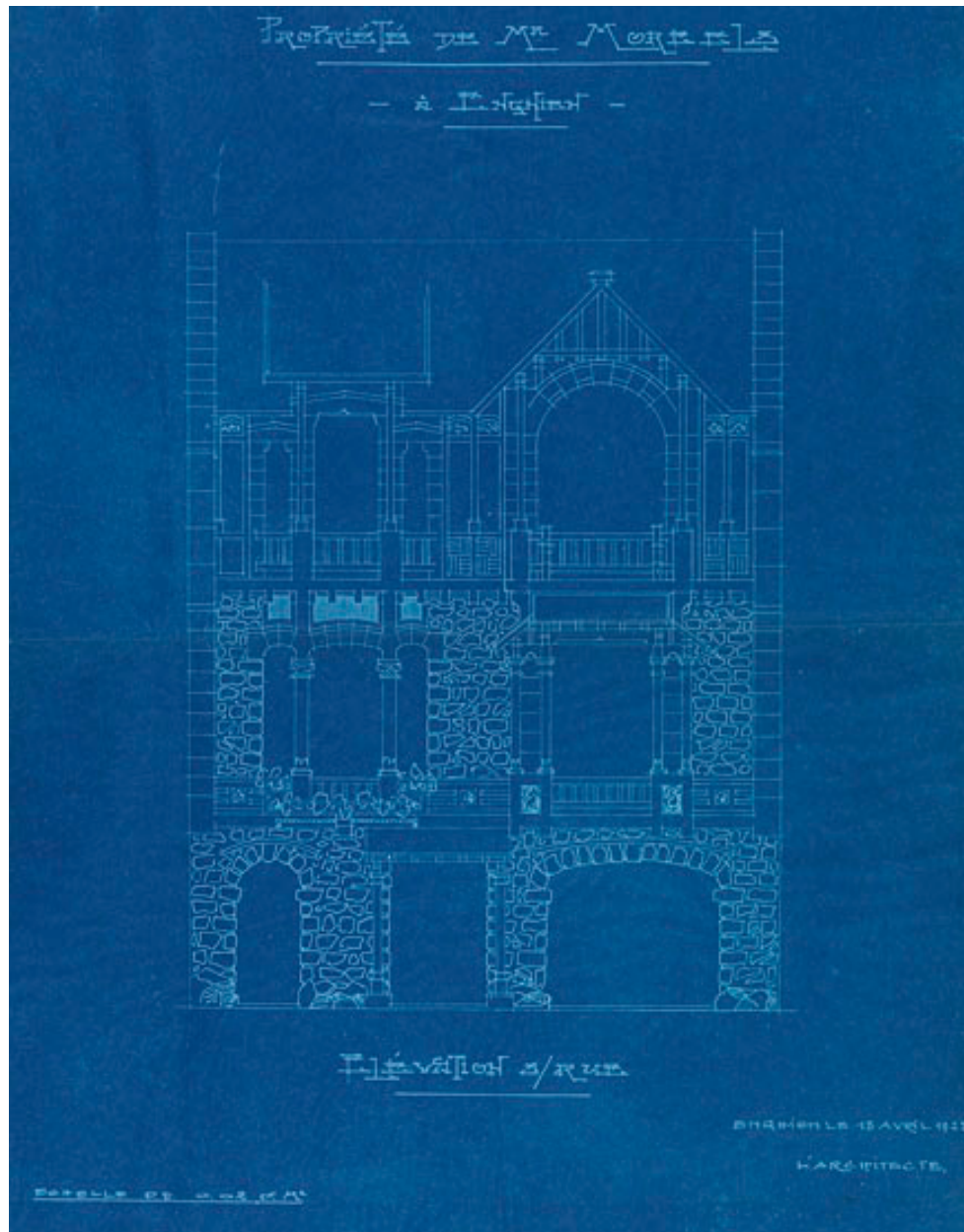
Elévation sur rue, 1922. (AM Enghien-les-Bains, 1T 194)
