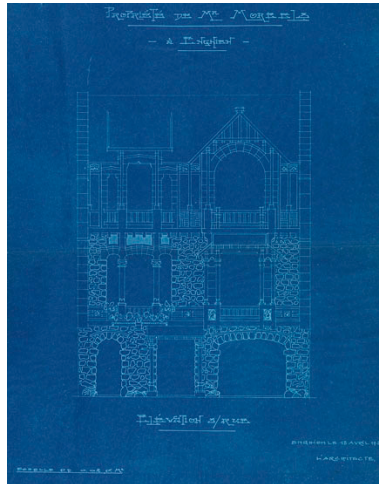
Elévation sur rue, 1922. (AM Enghien-les-Bains, 1T 194) Phot. Jean-Bernard Vialles, Autr. Henri (architecte) Moreels IVR11_20099500538NUC4A
