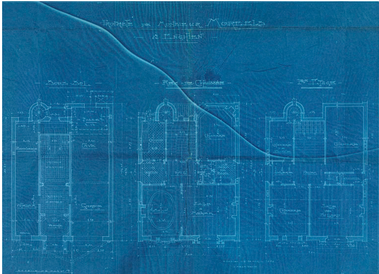
Plan des sous-sol, rez-de-chaussée et premier étage, 1922. (AM Enghien-les-Bains, 1T 194)
