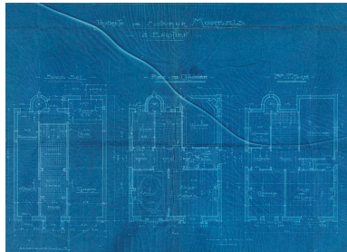
Plan des sous-sol, rez-de-chaussée et premier étage, 1922. (AM Enghien-les-Bains, 1T 194) Phot. Jean-Bernard Vialles, Autr. Henri (architecte) Moreels IVR11_20099500537NUC4A
