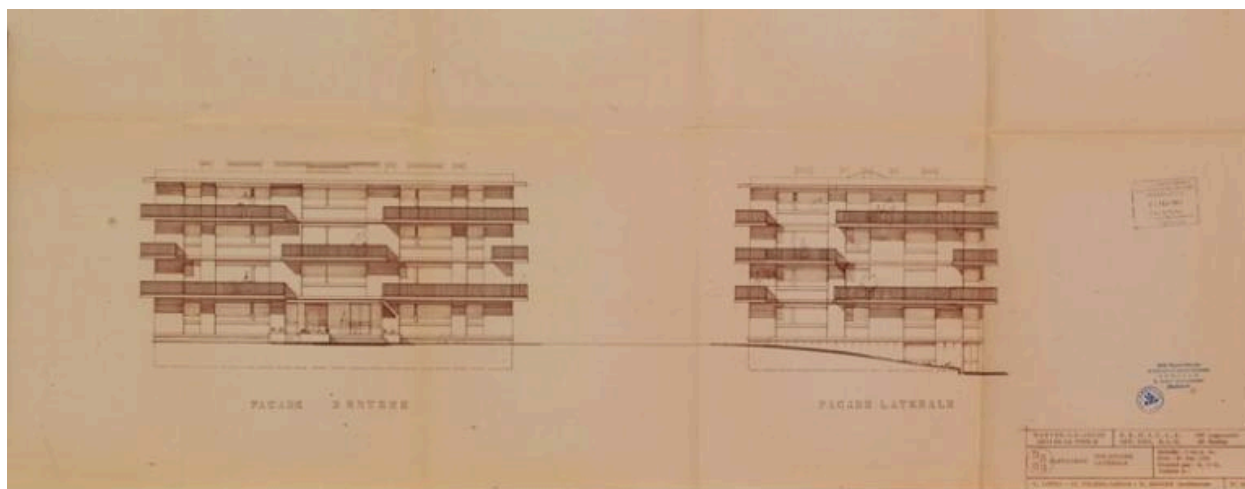
Façades des immeubles plots de la résidence Saint-Maclou. Mantes-la-Jolie. Permis de construire 4/68
