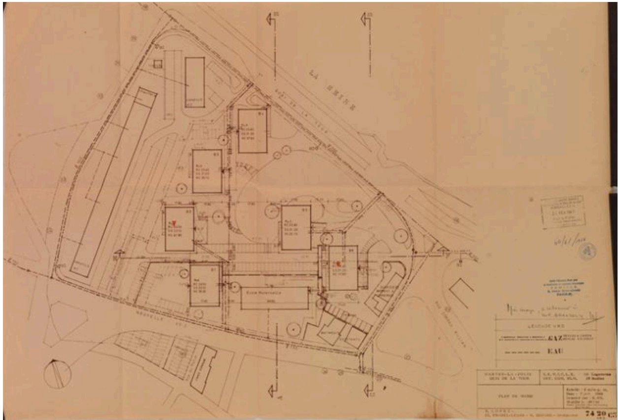
Plan masse de la résidence Saint-Maclou en mars 1966, 6 immeubles et des bâtiments à conserver. Mantes-la-Jolie. Permis de construire 61-61/66
