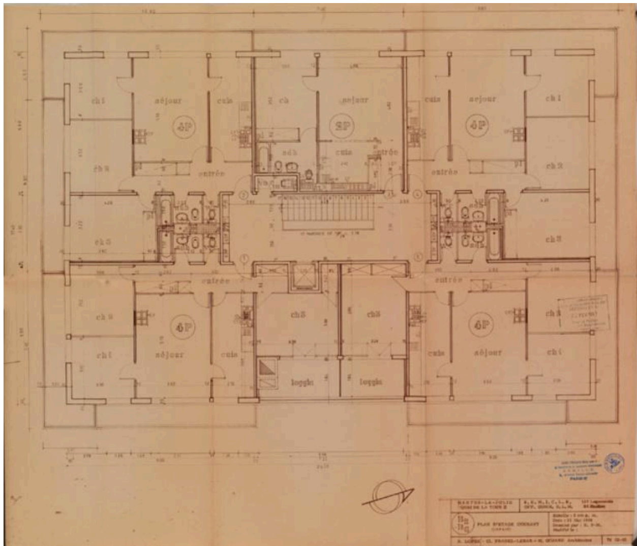
Plan d'un étage courant des immeubles de la résidence Saint-Maclou, 1966. Mantes-la-Jolie. Permis de construire 60-61/66
