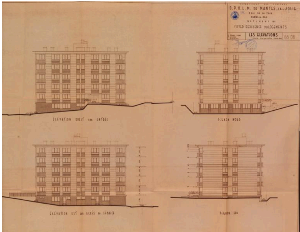
Façades de la résidence pour personnes âgées projetée en 1968. Mantes-la-Jolie. Permis de construire 60-61/66
