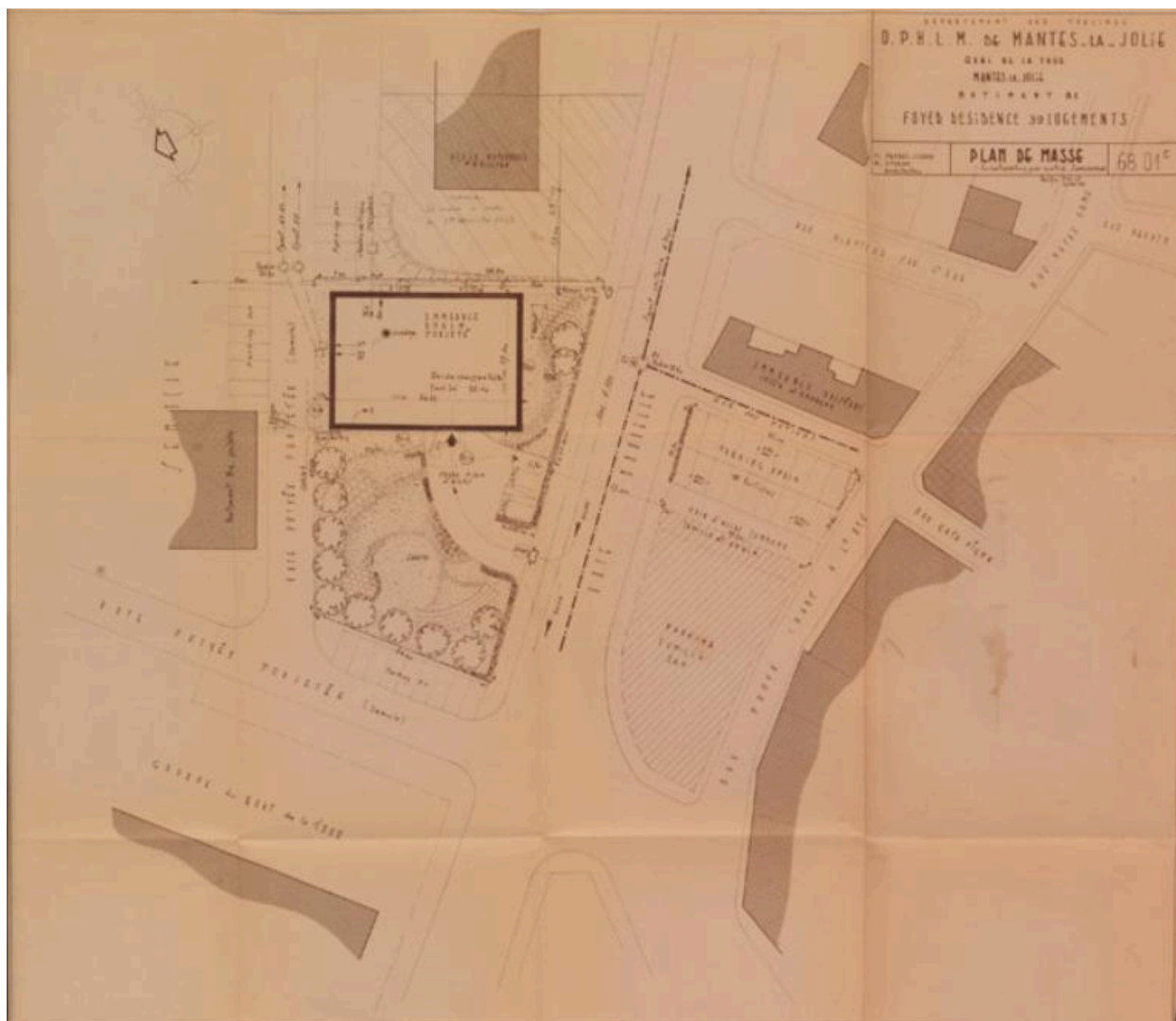
Plan masse de la résidence pour personnes âgées projetée en 1968. Mantes-la-Jolie. Permis de construire 60-61/66
