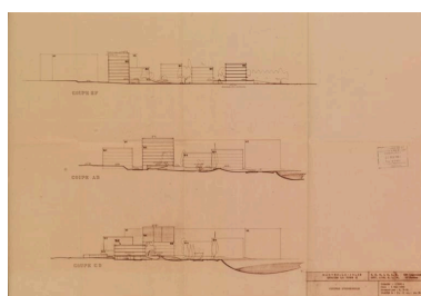
Coupes sur la résidence Saint-Maclou. On voit la volonté de respecter des cônes de vue. Mantes-la-Jolie. Permis de construire 60-61/66
