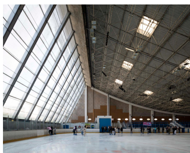
Vue générale de la verrière, qui éclaire de manière latérale la patinoire. Phot. Philippe Ayrault IVR11_20229100744NUC4A
