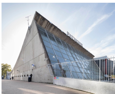
Vue générale de la verrière depuis l'allée de l'Agora. Phot. Philippe Ayrault IVR11_20229100755NUC4A
