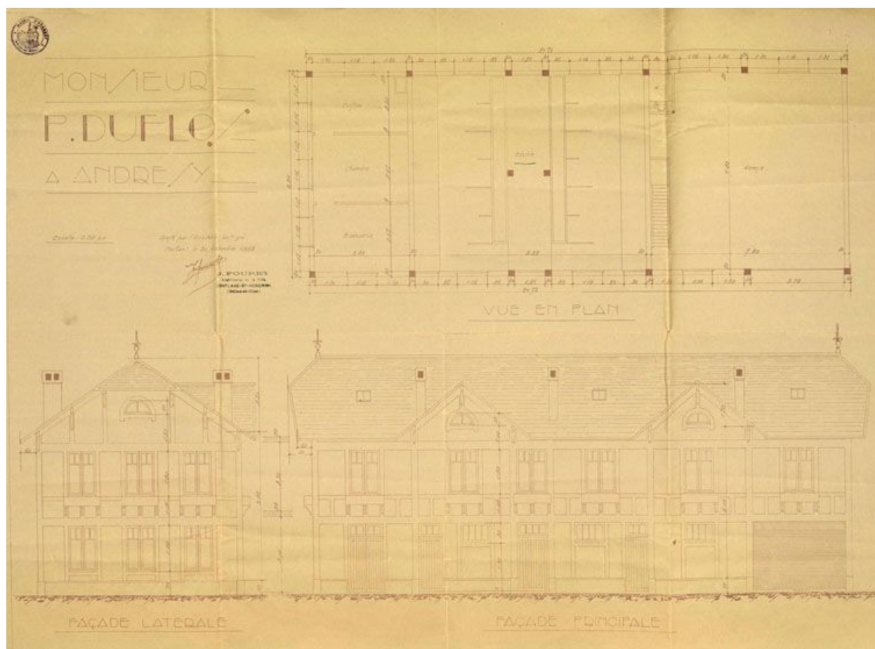
Projet de bâtiment agricole. Plan réalisé par Fouret pour Duflos. (AD Yvelines, O Lotissements 3).
