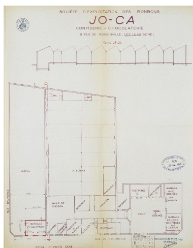
Plans accompagnant une demande de permis de construire : plan-masse et coupe N-S de l'ensemble de l'usine, emplacement de la "nouvelle chaufferie", 1948. (Ville des Lilas, dossier Permis de construire 1948-1). IVR11_20059300376XA
