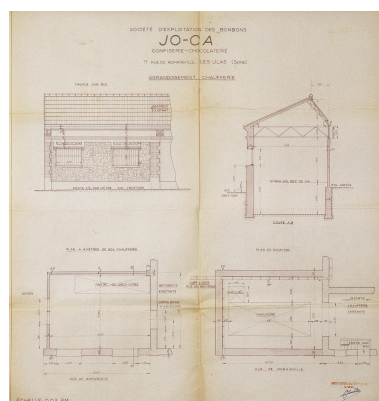
Plan accompagnant une demande de permis de construire : "Agrandissement chaufferie" (élévation et coupes), 1948. (Ville des Lilas, dossier Permis de construire 1948-1). IVR11_20059300377XA
