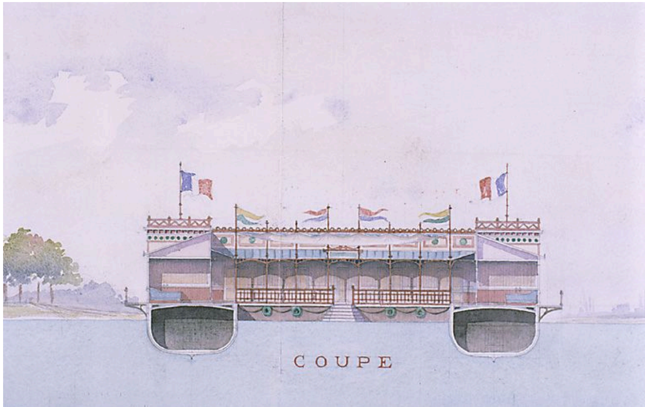
Projet d'installation en Seine sur la rive de Draveil d'un établissement de bains-douches, d'un lavoir et d'un bassin de natation : coupe transversale montrant la structure flottante et l'alimentation du bassin en eau de rivière, planche aquarellée, datée 1893 et signée L. Ducastel. (AD Essonne, 3 S 26)
