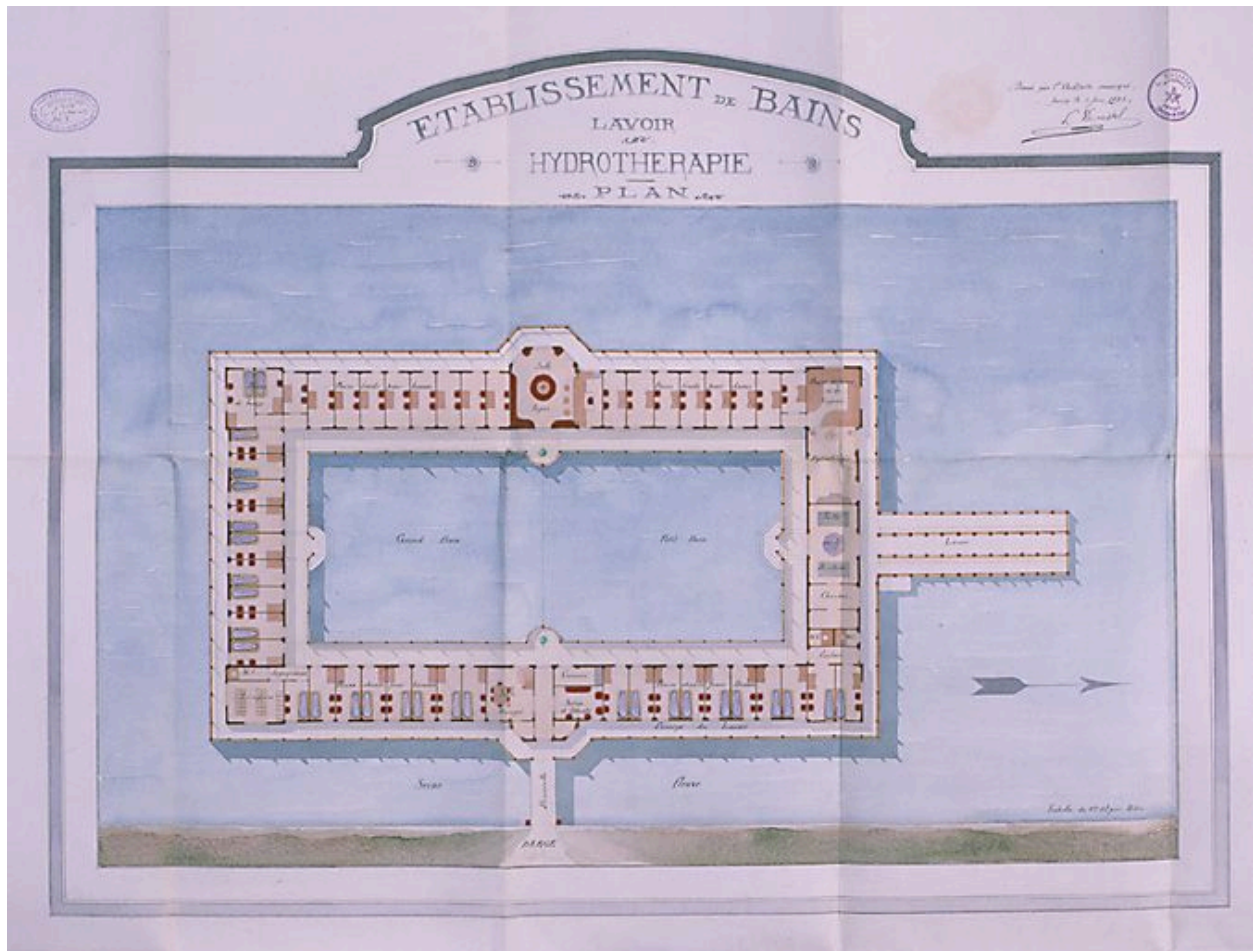
Projet d'installation en Seine d'un établissement de bains-douches, d'un lavoir et d'un bassin de natation : plan général, planche aquarellée, datée 1893 et signée L. Ducastel. (AD Essonne, 3 S 26)
