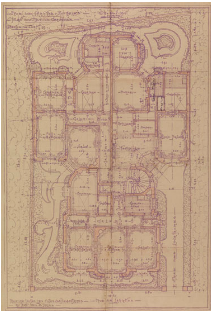
Plan du rez-de-chaussée (1908). (AM Enghien-les-Bains, 1T 8)
