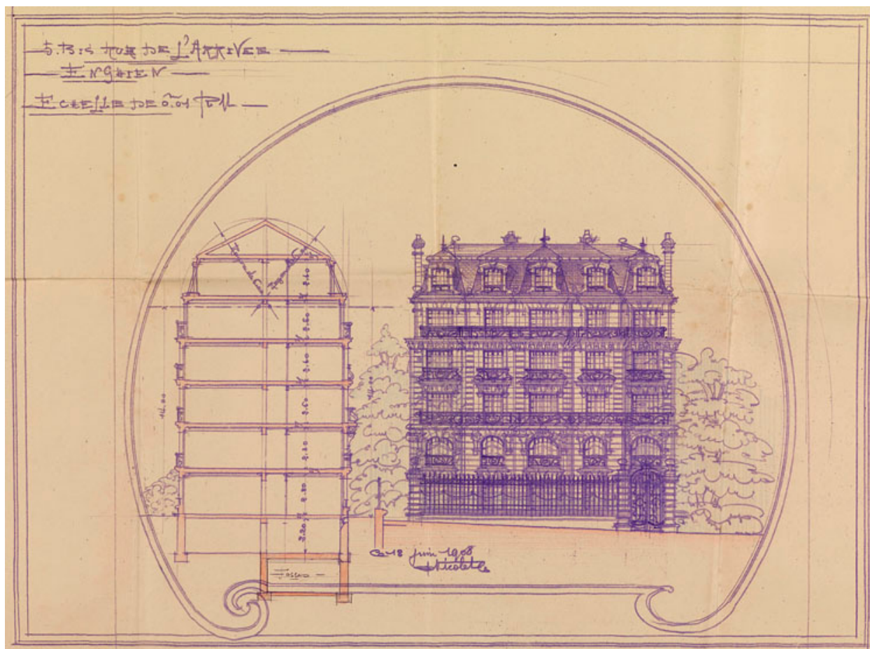
Coupe et élévation sur rue de l'immeuble (18 juin 1908) (AM Enghien-les-Bains, 1T 8)
