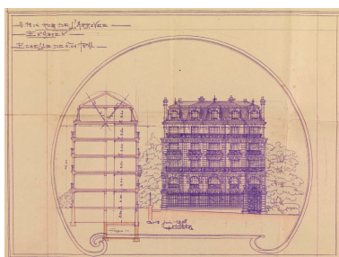
Coupe et élévation sur rue de l'immeuble (18 juin 1908) (AM Enghien-les-Bains, 1T 8) Phot. Jean-Bernard Vialles, Autr. Léon (architecte) Nicolet IVR11_20099500205NUC4A
