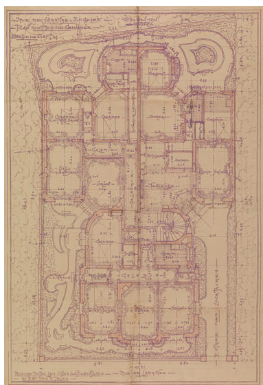
Plan du rez-de-chaussée (1908). (AM Enghien-les-Bains, 1T 8) Phot. Jean-Bernard Vialles, Autr. Léon (architecte) Nicolet IVR11_20099500207NUC4A
