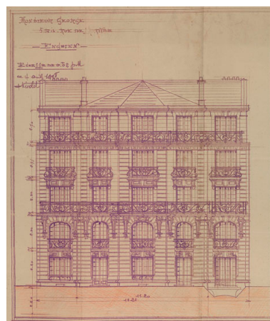
Premier projet d'élévation sur rue de l'immeuble alors dépourvu d'étage de comble (avril 1908) (AM Enghien-les-Bains, 1T 8) Phot. Jean-Bernard Vialles, Autr. Léon (architecte) Nicolet IVR11_20099500206NUC4A
