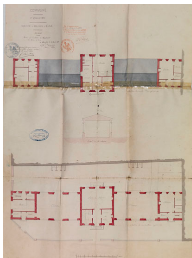
Plans du rez-de-chaussée et du premier étage par l'architecte départemental Blondel, 1863. Dessin aquarellé. (AM Enghien-les-Bains, M2) Phot. Jean-Bernard Vialles, Autr. Blondel (architecte) IVR11_20099500069NUC4A
