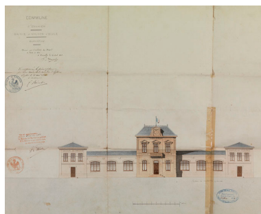
Elévation par l'architecte départemental Blondel, 1863. Dessin aquarellé, 1863. (AM Enghien-les-Bains, M2) Phot. Jean-Bernard Vialles, Autr. Blondel (architecte) IVR11_20099500070NUC4A
