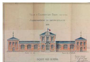
Elévation de la façade rue de Mora, exécutée à l'occasion de l'agrandissement du groupe scolaire lors du départ des services de la mairie dans de nouveaux locaux, 1894. Dessin aquarellé. (AM Enghien-les-Bains, M2) Phot. Jean-Bernard Vialles, Autr. A. (architecte) Vernholes IVR11_20099500071NUC4A
