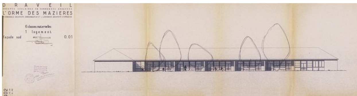
Bâtiment comprenant six classes maternelles et un logement d'instituteurs : plan de la façade sud. (AD Essonne, 1051 W 29-30)
