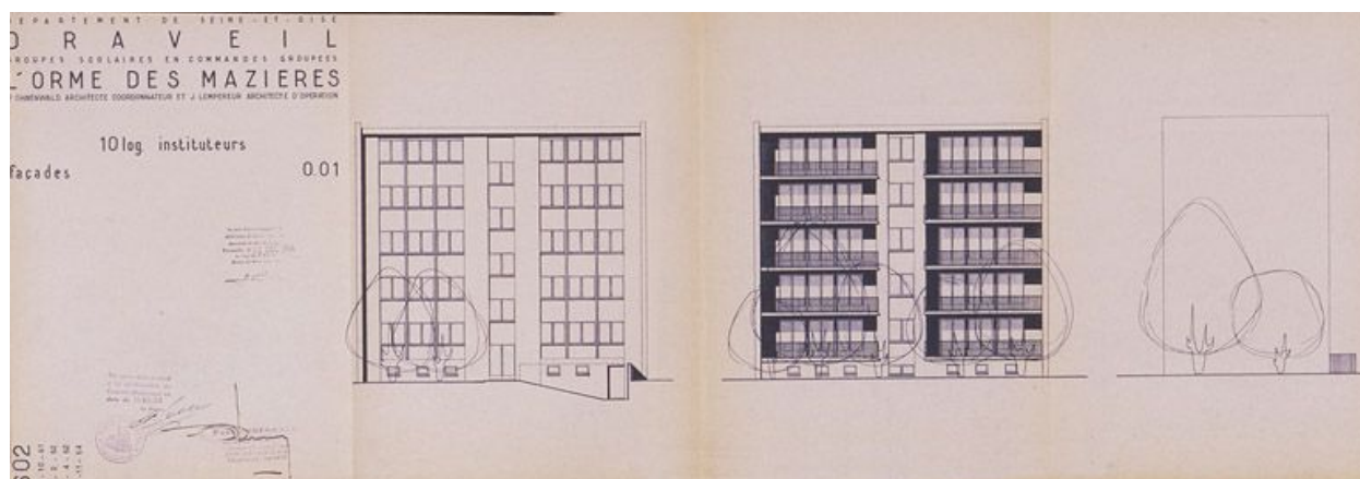
Bâtiment comprenant 10 logements d'instituteurs : plans des façades. (AD Essonne, 1051 W 29-30)
