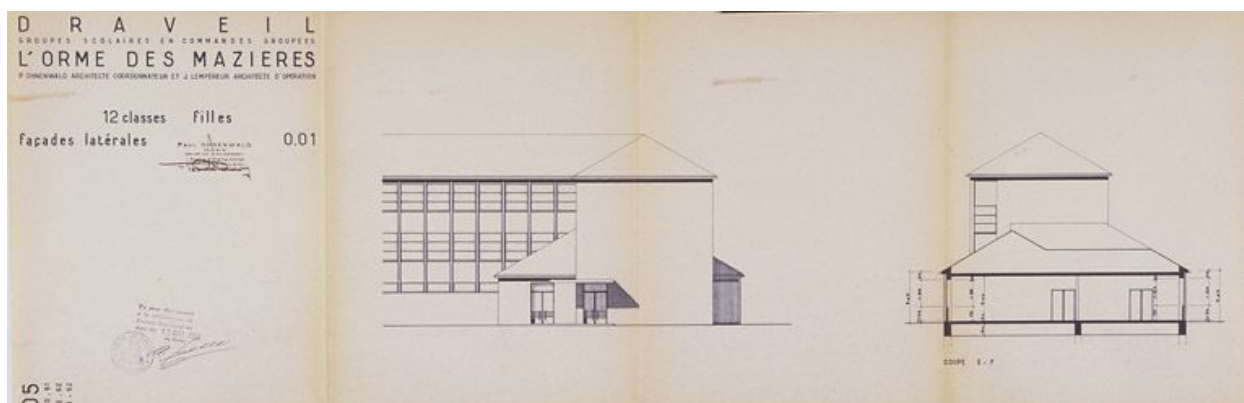
Ecole des filles (douze classes) : plan des façades latérales. (AD Essonne, 1051 W 29-30)
