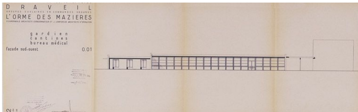
Bâtiment comprenant le bureau du gardien, les cantines et le bureau médical : plan de la façade sud-ouest. (AD Essonne, 1051 W 29-30)
