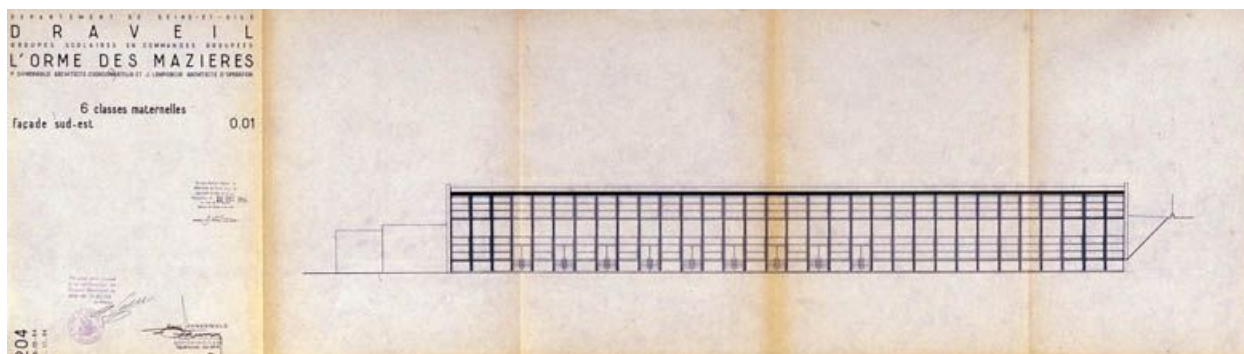
Bâtiment de la maternelle (six classes), plan de la façade sud-est. (AD Essonne, 1051 W 29-30)
