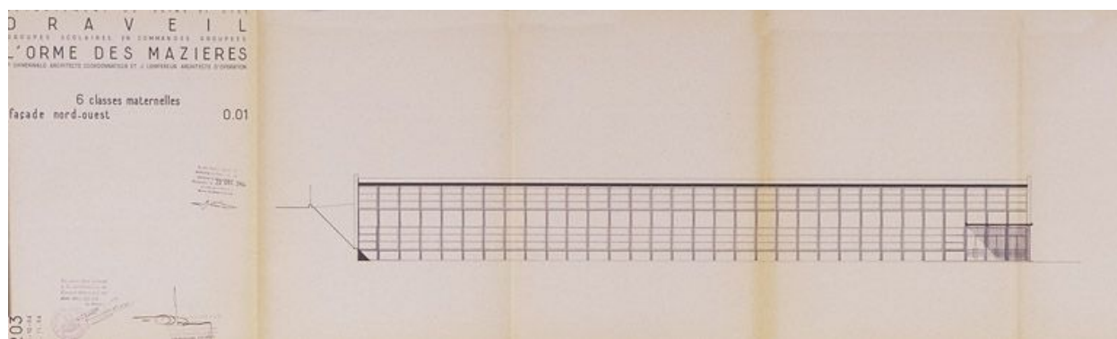
Bâtiment de la maternelle (six classes) : plan de la façade nord-ouest. (AD Essonne, 1051 W 29-30)
