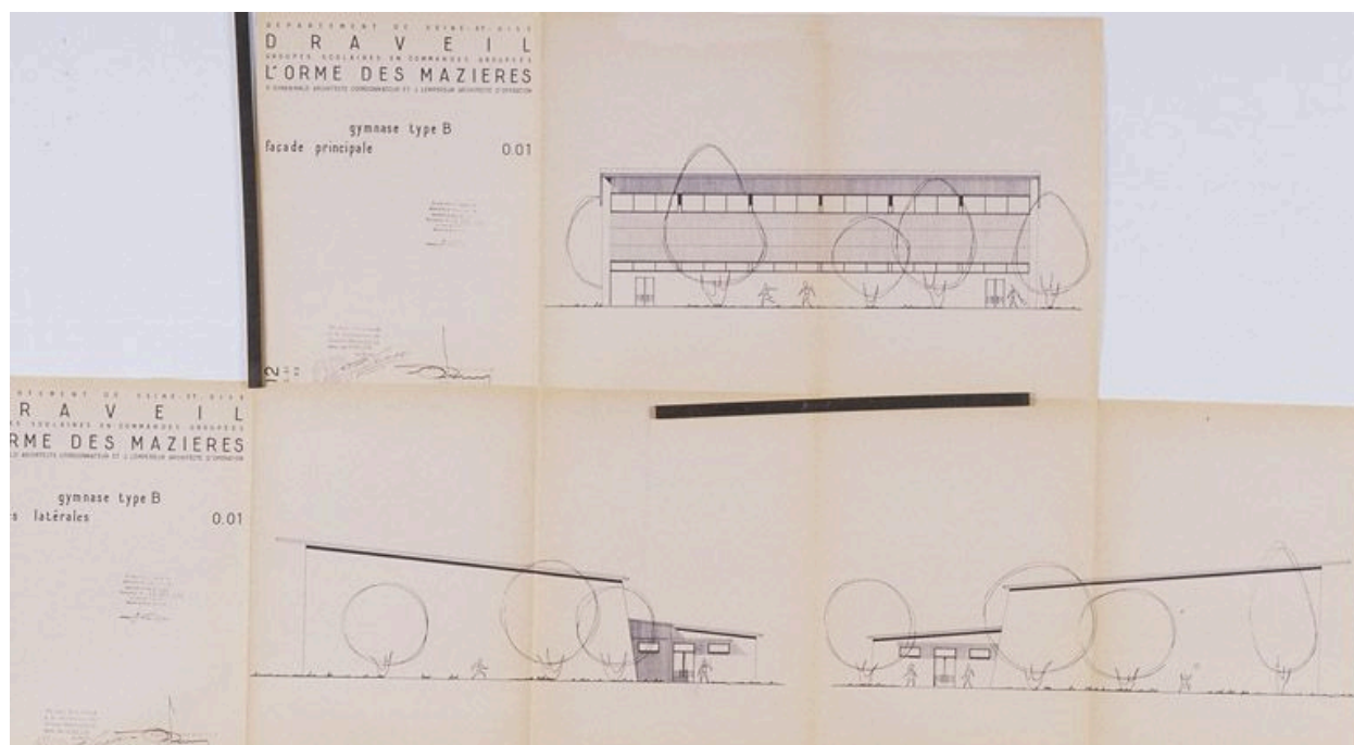
Gymnase type B : plans des façades principale et latérales. (AD Essonne, 1051 W 29-30)
