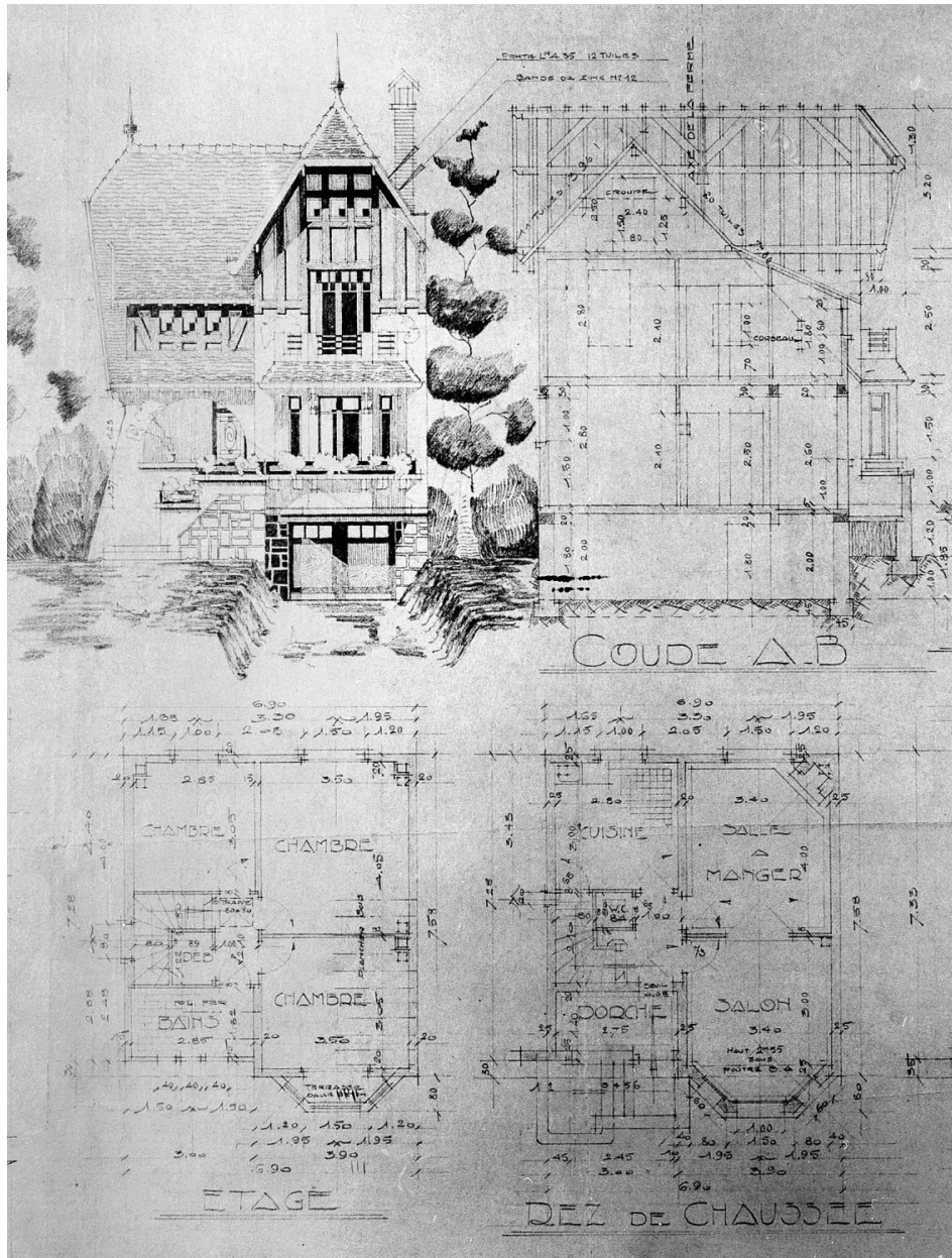
Elévation, plans et coupe.
