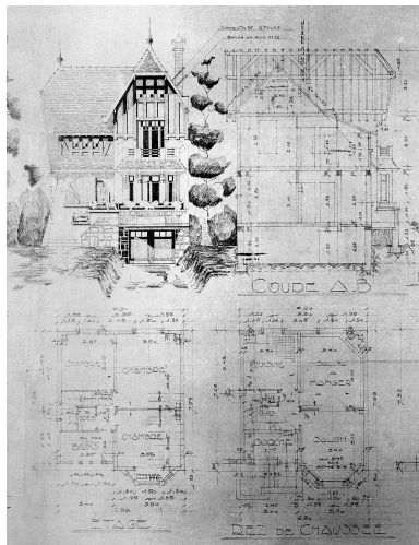
Elévation, plans et coupe. IVR11_20007800071X
