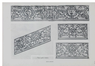
Modèle de panneaux rampants et paliers de la rampe en ferronnerie de style rocaille (Nancy, Intendance). Gravure, 18e siècle. Tiré de : Le fer forgé en France, la Régence : aurore, apogée, déclin, oeuvres gravées des anciens maîtres serruriers, architectes, dessinateurs et graveurs / Louis Blanc. Paris : G. Van Oest, 1930. Autr. Jean (serrurier) Lamour IVR11_20097501503NUC4A
