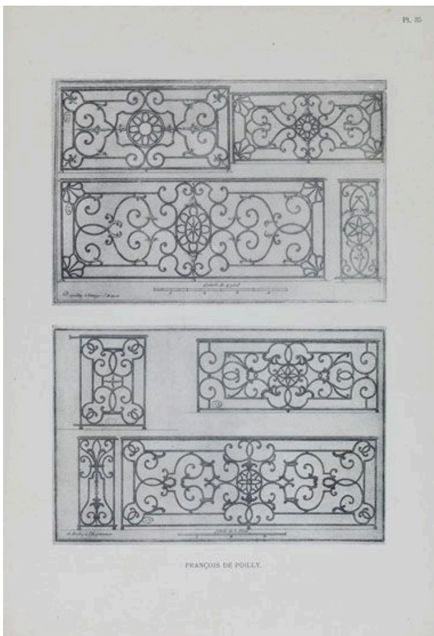
Modèles de panneaux droits et de pilastres (non localisé). Gravure, 18e siècle. Tiré de : Le fer forgé en France aux XVIe et XVIIe siècles, oeuvres gravées des anciens maîtres serruriers, architectes, dessinateurs et graveurs / Louis Blanc. Paris : G. Van Oest, 1928.
