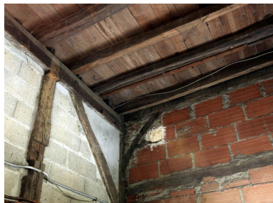
Atelier de charpentier, détail de l'architecture en pan de bois.
