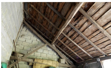
Appentis, détail de la charpente.
