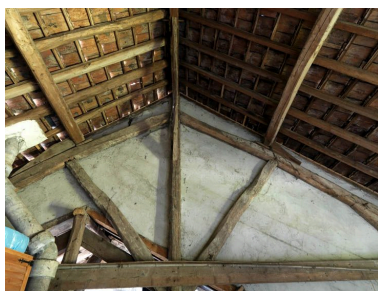
Charpente de l'atelier.
