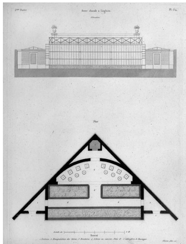
Plan et élévation d'une serre chaude. Gravure. (BHVP, in fol. 10 84) Phot. Bernard Emmanuelli IVR11_19697500454P
