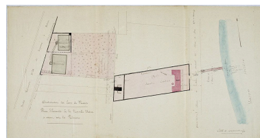
L'usine des eaux (disparue) : plan d'ensemble, 1885. Calque aquarellé. (AD Seine-et-Marne. 4 Op 284/14) Phot. Yvan Bourhis IVR11_20137700031NUC4A
