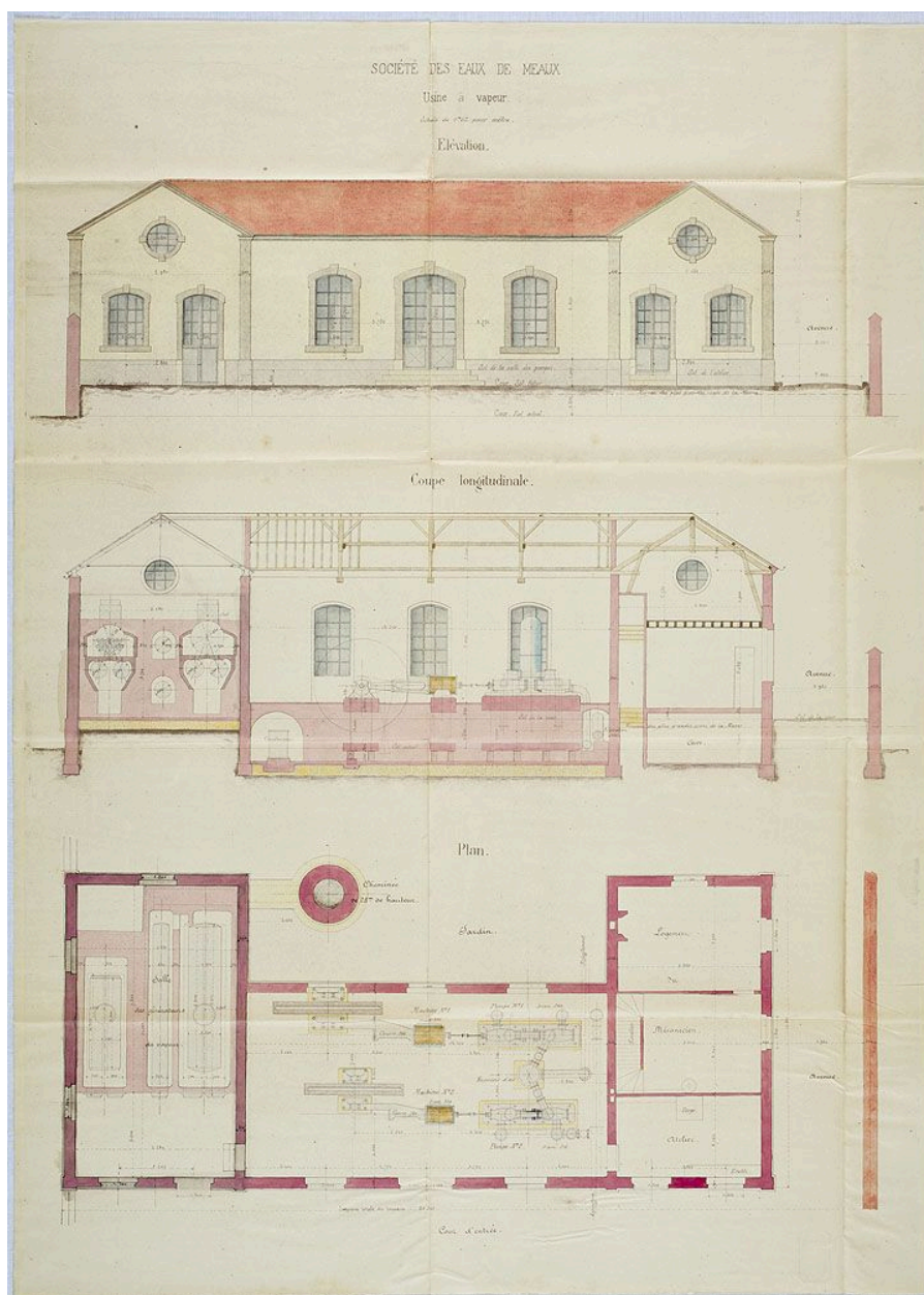
L'usine des eaux (disparue) : bâtiments de la nouvelle usine hydraulique à vapeur (1 élévation, 1 coupe, 1 plan), 1885. Calque aquarellé. (AD Seine-et-Marne. 4 Op 284/14)
