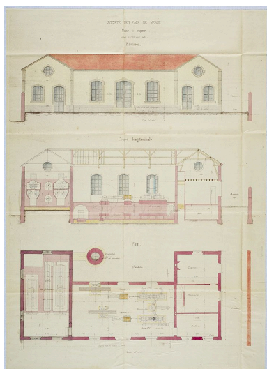
L'usine des eaux (disparue) : bâtiments de la nouvelle usine hydraulique à vapeur (1 élévation, 1 coupe, 1 plan), 1885. Calque aquarellé. (AD Seine-et-Marne. 4 Op 284/14) Phot. Yvan Bourhis IVR11_20137700032NUC4A
