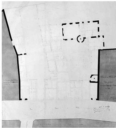
Album de 11 planches : projet d'hôtel de ville. Planche 1 : plan général des anciens bâtiments de l'hôtel de ville. Papier aquarellé, 1844. (BM Melun. JJ 9) Phot. Philippe Ayrault, Autr. Gilson (architecte de la ville) IVR11_20027701158X
