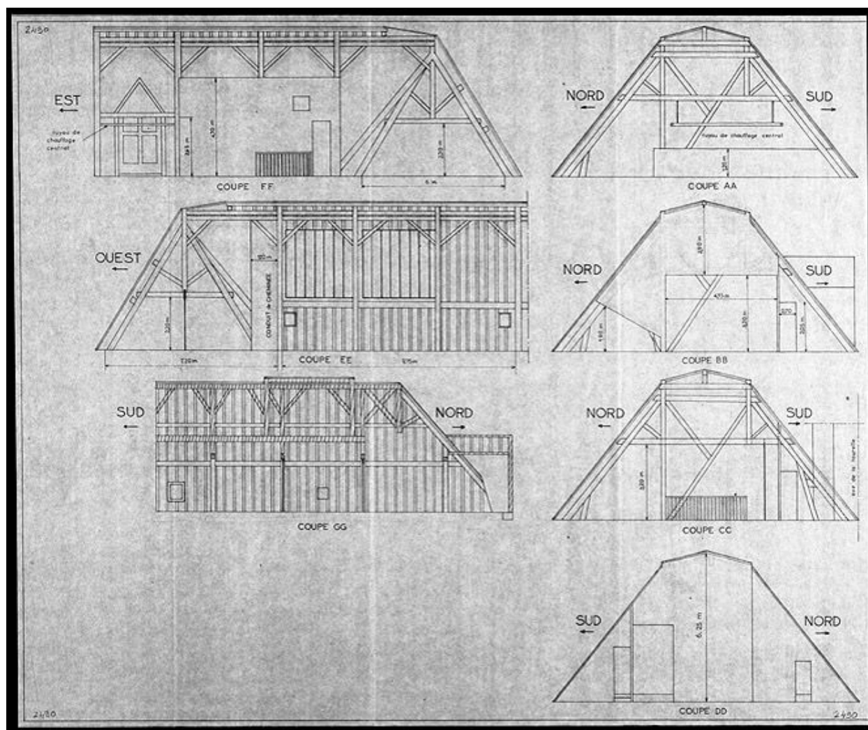
Hôtel de ville : grenier, partie ouest. Papier, tirage d'architecte, 1977. (AM Melun. 1 Fi 2490)
