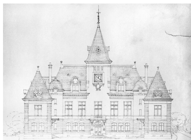
Projet non réalisé d'agrandissement de l'hôtel de ville : la façade. Papier, 1912 (vers). (AM Melun. 1 Fi 877)
