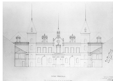
Album de 11 planches : projet d'hôtel de ville. Planche 8 : façade principale. Papier aquarellé, 1844. (BM Melun. JJ 9) Phot. Philippe Ayrault, Autr. Gilson (architecte de la ville) IVR11_20027701165X
