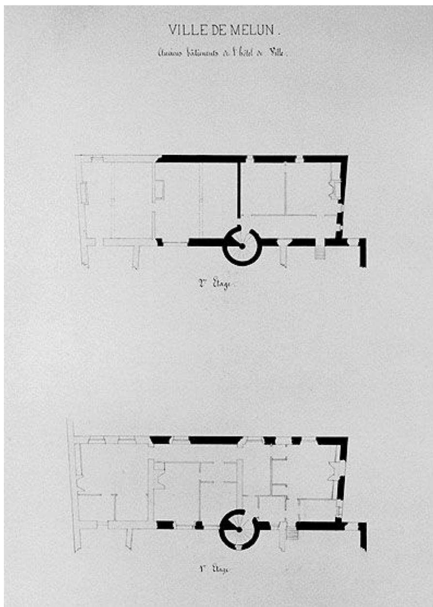
Album de 11 planches : projet d'hôtel de ville. Planche 2 : anciens bâtiments de l'hôtel de ville : grand bâtiment Dolibon. Plans du premier et deuxième étages. Papier aquarellé, 1844. (BM Melun. JJ 9)
