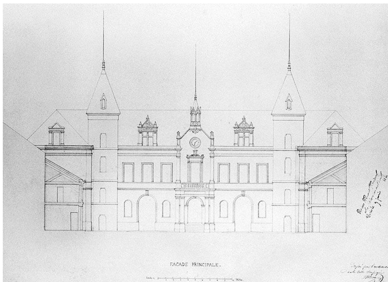
Album de 11 planches : projet d'hôtel de ville. Planche 8 : façade principale. Papier aquarellé, 1844. (BM Melun. JJ 9)
