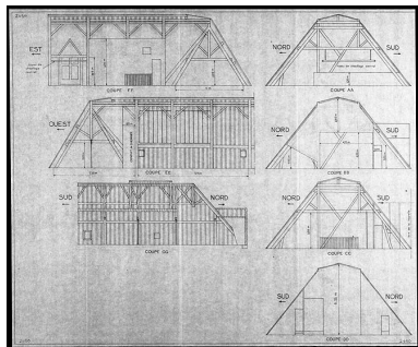
Hôtel de ville : grenier, partie ouest. Papier, tirage d'architecte, 1977. (AM Melun. 1 Fi 2490) Phot. Archives municipales de Melun (reproduction) IVR11_20047700553NUC
