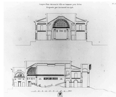
Coupes d'une Maison de Ville ou commune pour Melun proposée par Normand en 1793. Projet non réalisé. (BNF, Département des estampes. Est. Hd 78 pet. fol., planche 16) Phot. Département des Estampes (reproduction) Bibliothèque nationale de France, Autr. Normand IVR11_20067700570NUC
