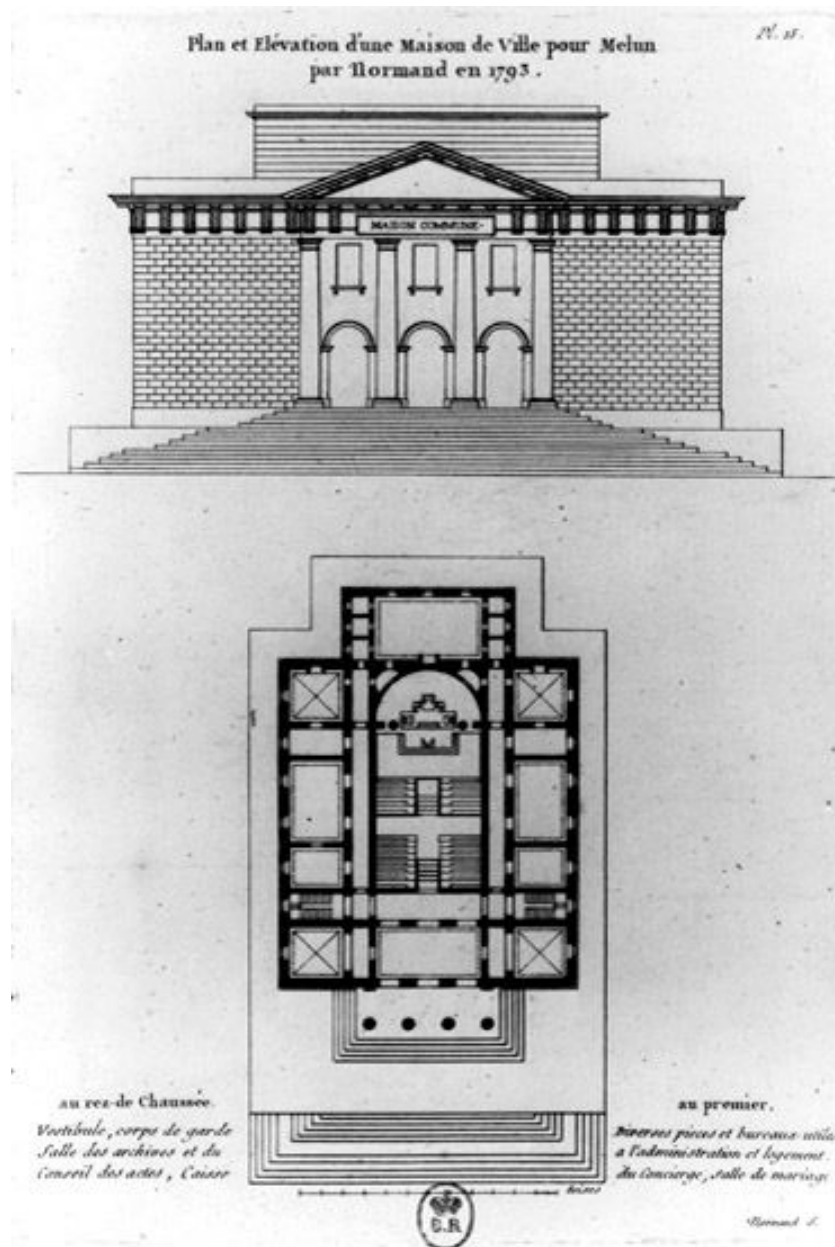
Plan et élévation d'une Maison de Ville pour Melun par Normand en 1793. Projet non réalisé. (BNF, Département des estampes. Est. Hd 78 pet. fol., planche 15)
