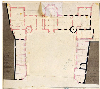
Album de 11 planches : projet d'hôtel de ville. Planche 6 : plan du rez-de-chaussée. Papier aquarellé, 1844. (BM Melun. JJ 9) Phot. Philippe Ayrault, Autr. Gilson (architecte de la ville) IVR11_20027701162XA
