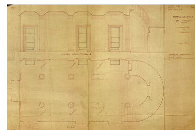
Hôtel de ville de Melun. Aménagement du vestibule. Papier, tirage d'architecte, 1946. (AM Melun. 1 Fi 2023)
