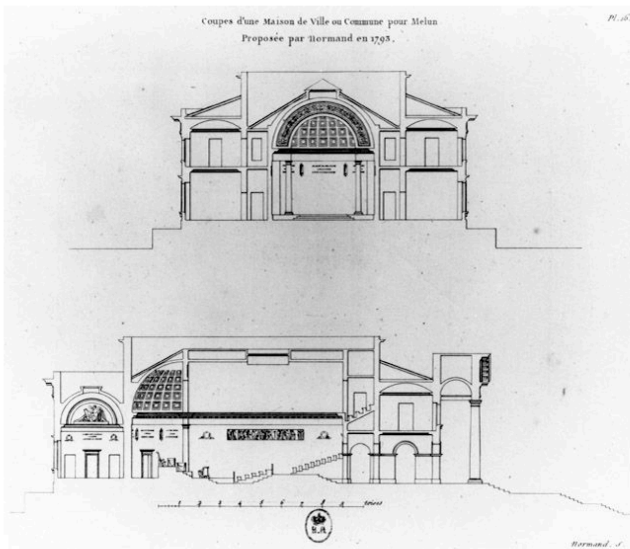
Coupes d'une Maison de Ville ou commune pour Melun proposée par Normand en 1793. Projet non réalisé. (BNF, Département des estampes. Est. Hd 78 pet. fol., planche 16)
