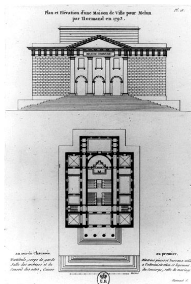
Plan et élévation d'une Maison de Ville pour Melun par Normand en 1793. Projet non réalisé. (BNF, Département des estampes. Est. Hd 78 pet. fol., planche 15) Phot. Département des Estampes (reproduction) Bibliothèque nationale de France, Autr. Normand IVR11_20067700569NUC
