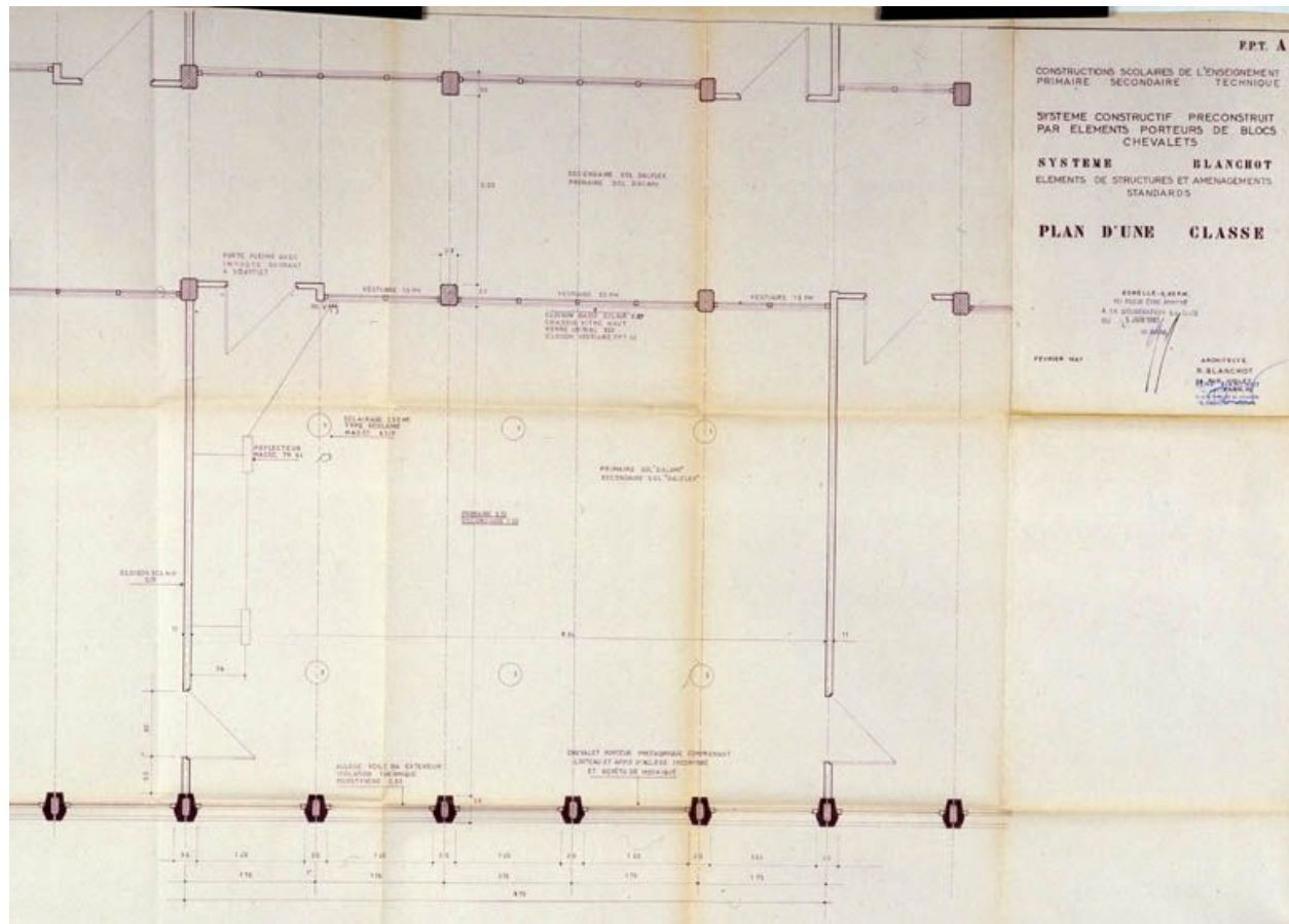
Plan d'une classe construite selon le système Blanchot (système constructif préconstruit par éléments porteurs de blocs chevalets, éléments de structures et aménagements standards). (AD Essonne, 1051 W 200)
