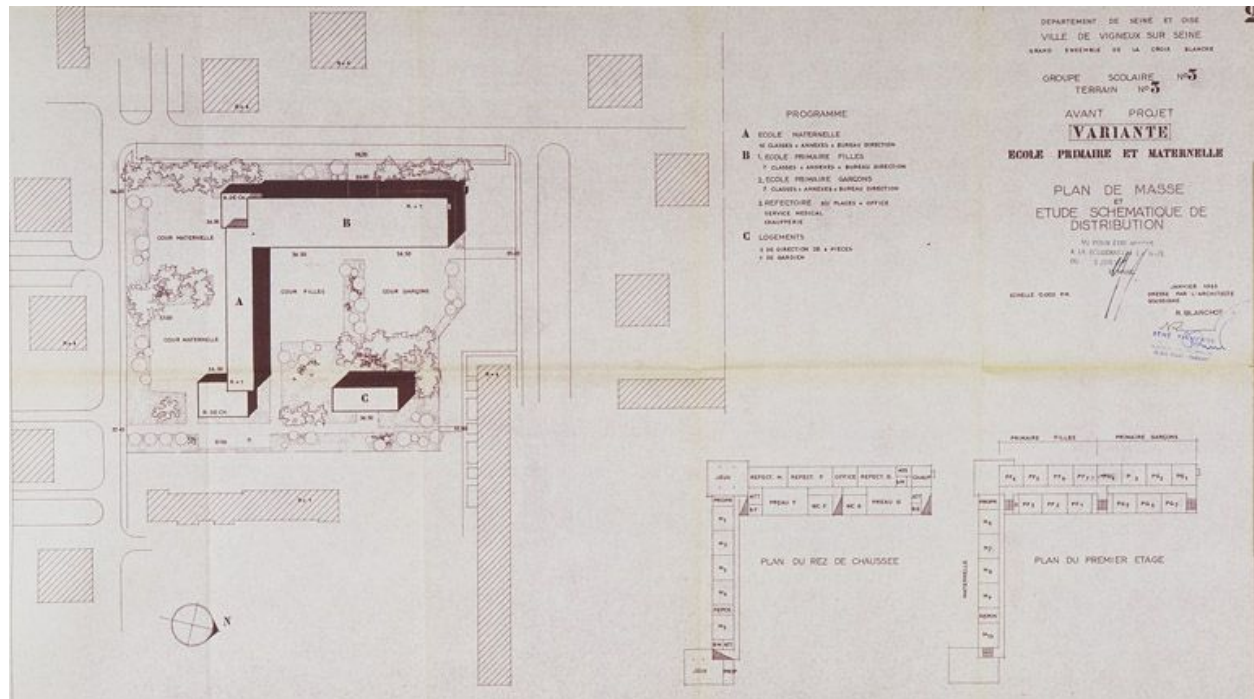
Avant-projet, variante : plan de masse et étude schématique de distribution. (AD Essonne, 1051 W 200)
