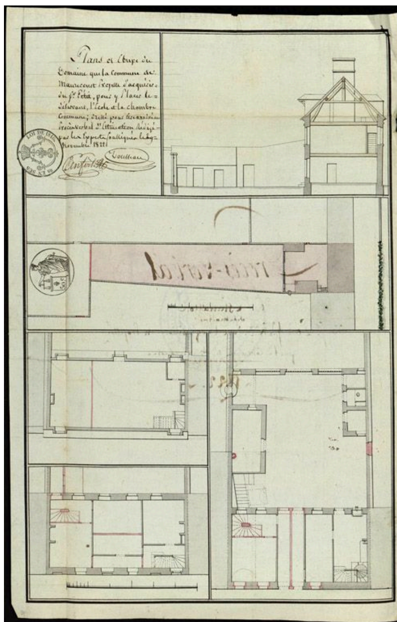
Plan et coupe du domaine que la commune de Maurecourt projette d'acquiescer...", 1822. Dessin. (AD Yvelines).
