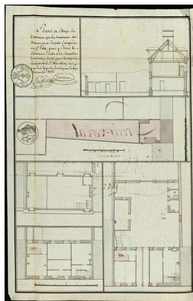
Plan et coupe du domaine que la commune de Maurecourt projette d'acquérir..., 1822.
