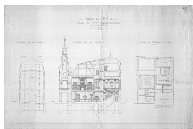
Plan de coupe de la Mairie du XIVe dressé par A-E Auburtin, 1881. (AD75 V27 M4 art.1-13). IVR11_20157500516NUC4A
