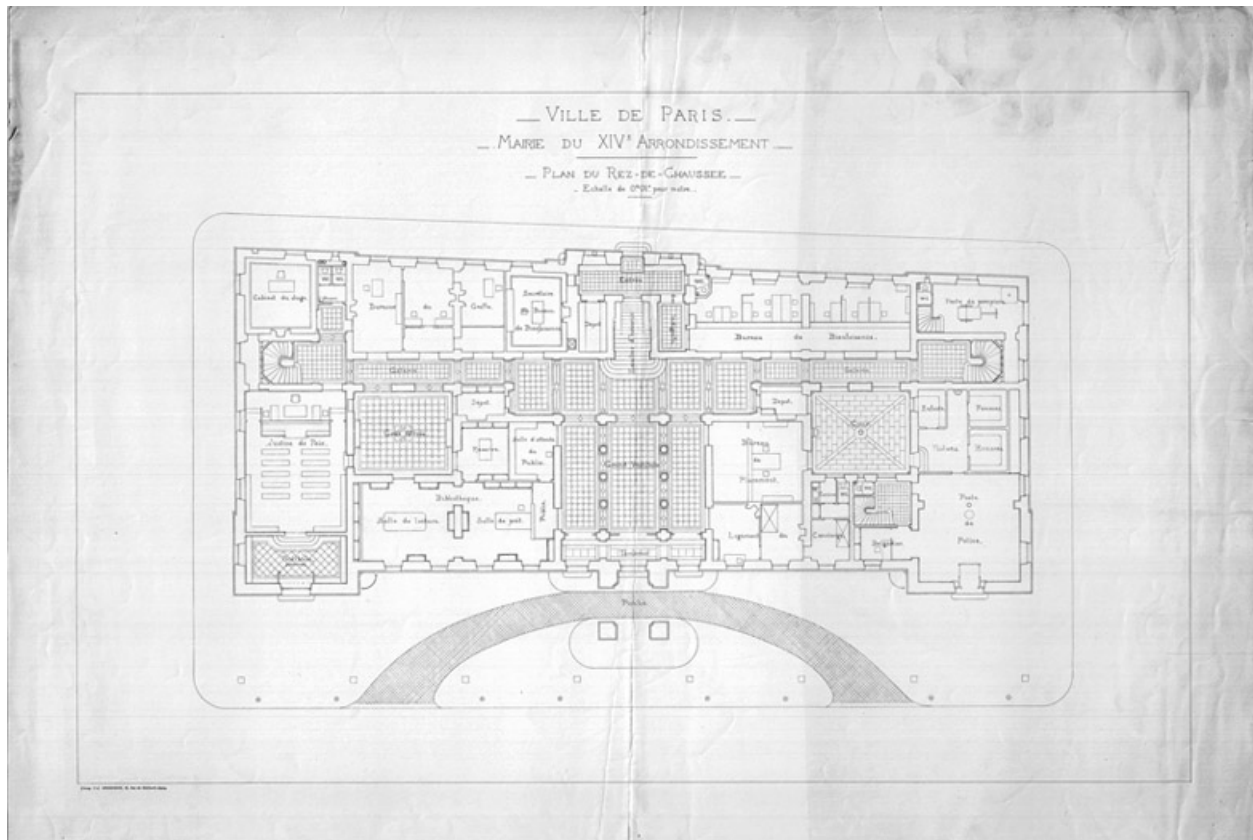
Plan du rez de chaussée de la Mairie du XIVe dressé par A-E Auburtin, 1881. (AD75 V27 M4 art.1-13).
