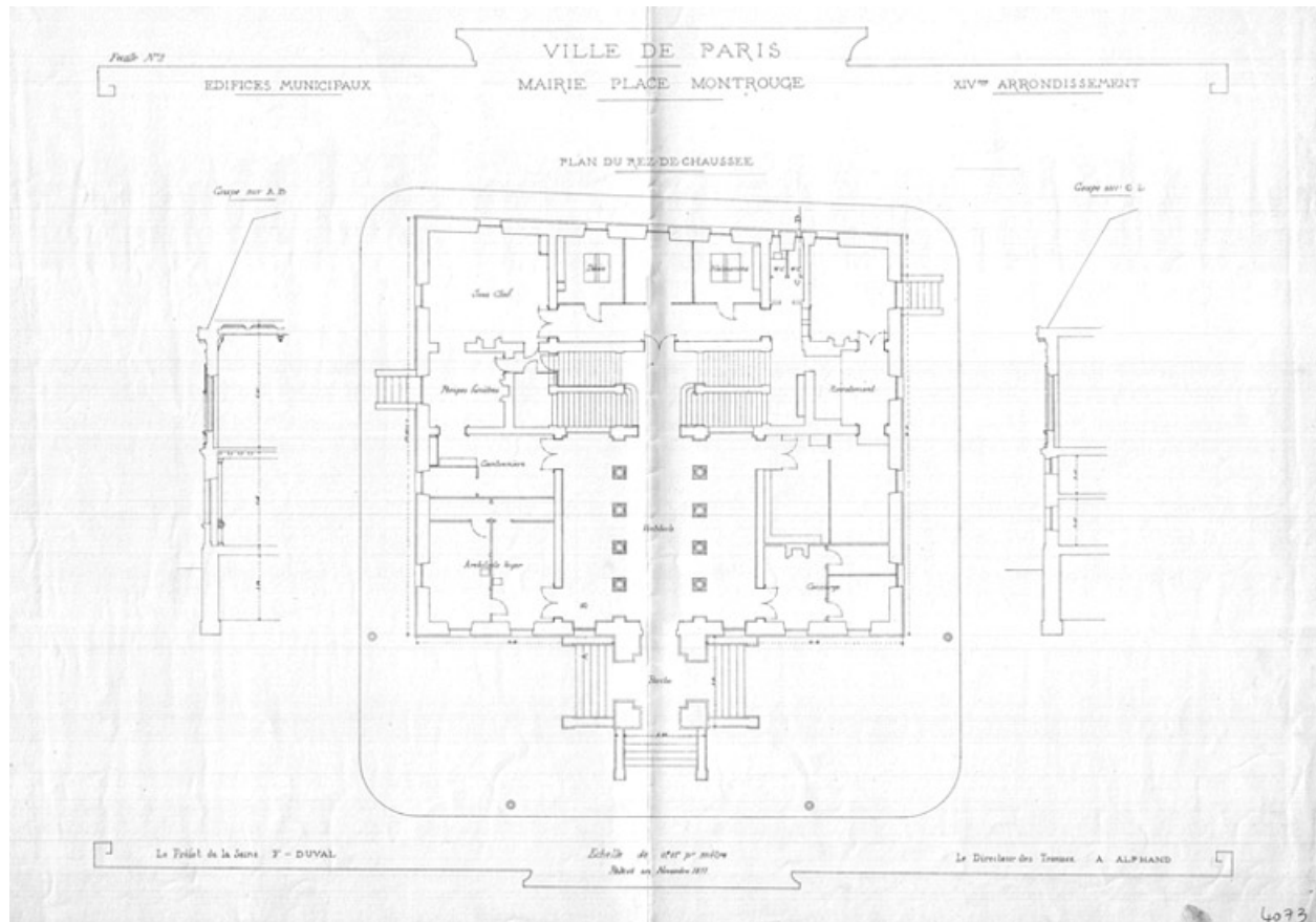
Plan du rez de chaussée de la Mairie Place de Montrouge relevé en 1877. (AD75. V27-M4 art.1-13)
