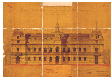
Projet d'agrandissement de la Mairie du XIVe, élévation principale, dressé par A-E Auburtin en 1881. (AD75 V27 M4 art.1-13)
