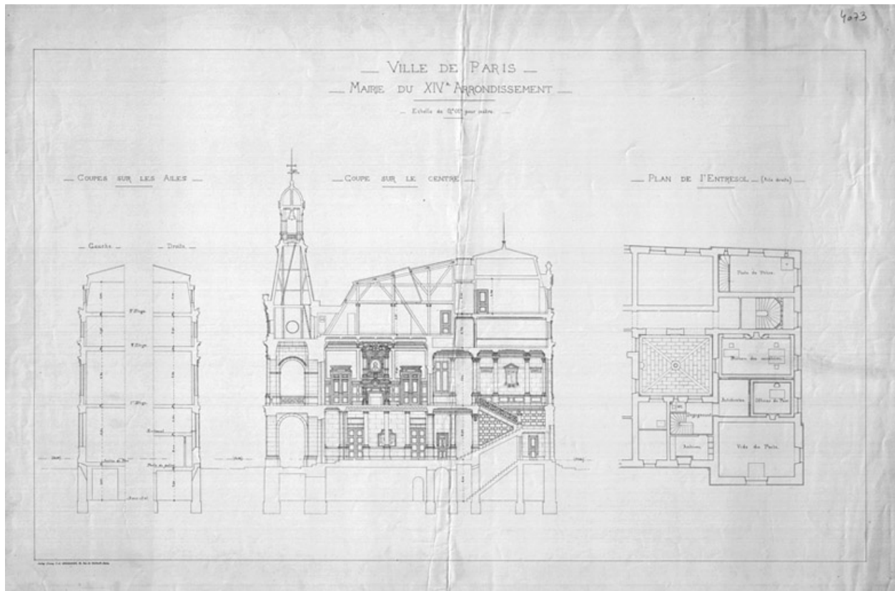
Plan de coupe de la Mairie du XIVe dressé par A-E Auburtin, 1881. (AD75 V27 M4 art.1-13).
