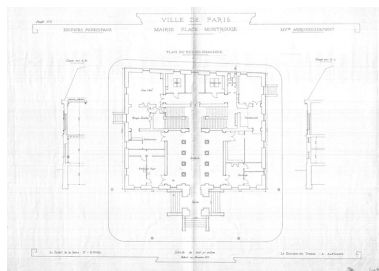
Plan du rez de chaussée de la Mairie Place de Montrouge relevé en 1877. (AD75. V27-M4 art.1-13) IVR11_20157500517NUC4A
