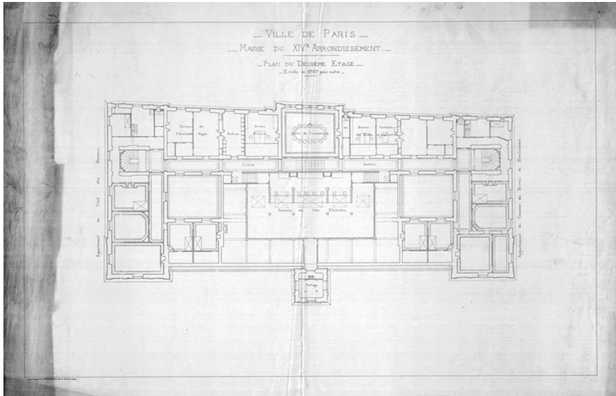
Plan du 2e étage de la Mairie du XIVe dressé par A-E Auburtin, 1881. (AD75 V27 M4 art.1-13).
