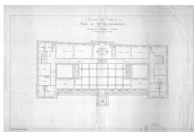
Plan du 3e étage de la Mairie du XIVe dressé par A-E Auburtin, 1881. (AD75 V27 M4 art.1-13). IVR11_20157500514NUC4A
