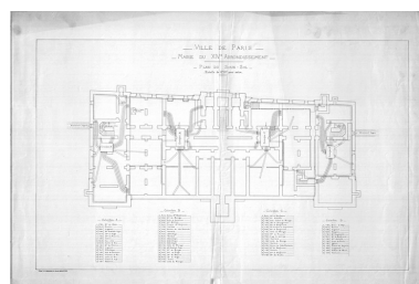
Plan du sous-sol de la Mairie du XIVe dressé par A-E Auburtin, 1881. (AD75 V27 M4 art.1-13). IVR11_20157500513NUC4A
