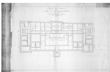
Plan du 2e étage de la Mairie du XIVe dressé par A-E Auburtin, 1881. (AD75 V27 M4 art.1-13). IVR11_20157500515NUC4A
