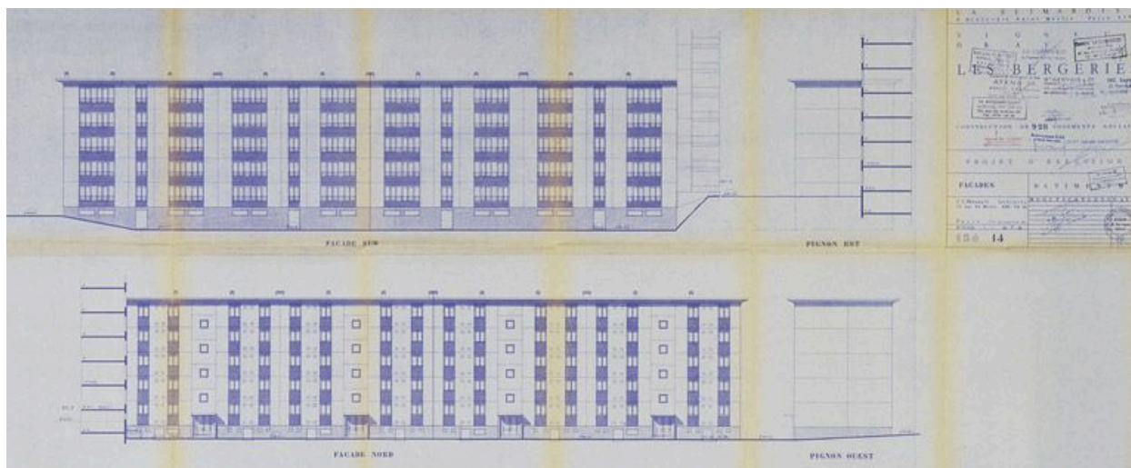
Construction de 928 logements sociaux : façades du bâtiment 9. (AD Essonne, 1502 W 1233)
