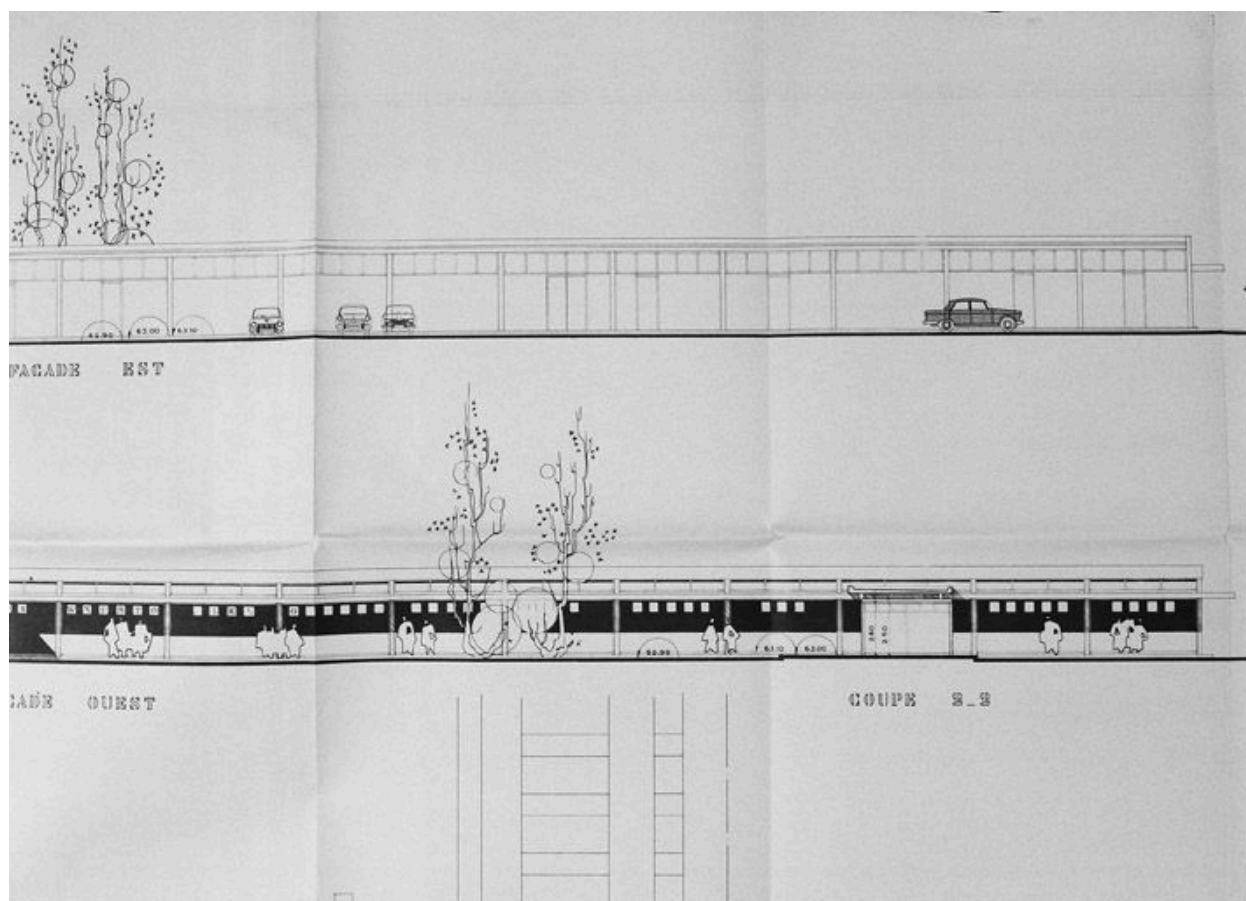
Centre commercial : détail des façades est et ouest ; plans dressés par J. L'Hernault, 1er janvier 1967. (AM Vigneux-sur-Seine, 80 W 31)
