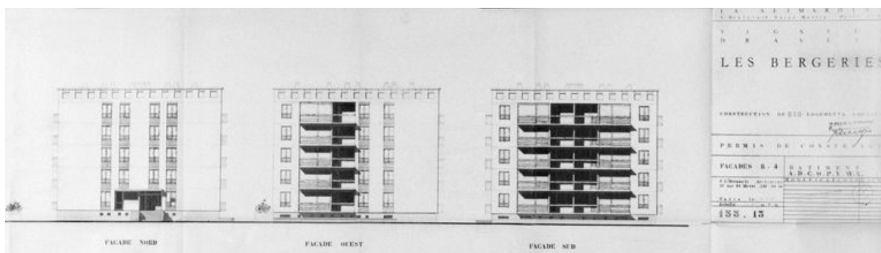
Bâtiments R + 4 (A, D, C, O, P, V, W et X) : plans des façades nord, ouest et sud, dressés par J. L'Hernault, 16 juillet 1965. (AM Vigneux-sur-Seine, 80 W 29, dossiers 57-58)
