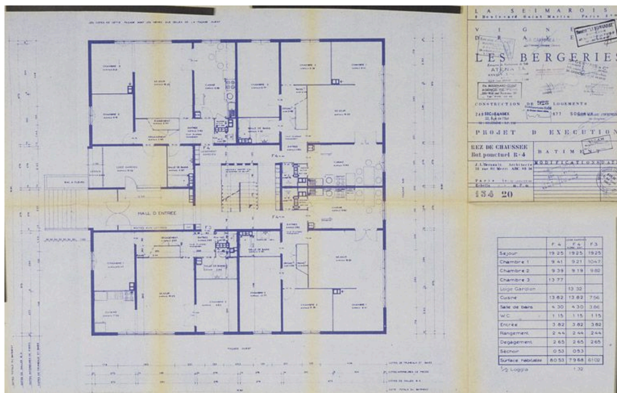
Construction de 928 logements sociaux : bâtiment ponctuel R + 4, plan du rez-de-chaussée. (AD Essonne, 1502 W 1233)
