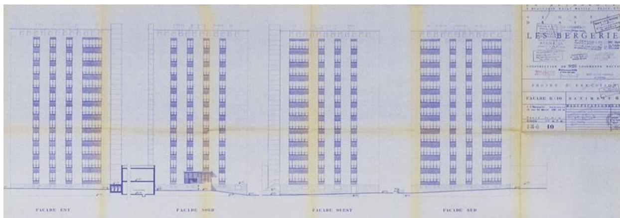
Construction de 928 logements sociaux : façades des bâtiments R +10. (AD Essonne, 1502 W 1233)
