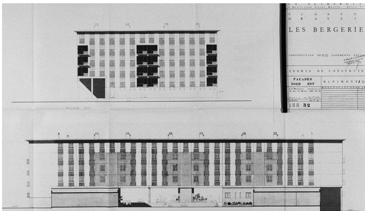
Bâtiment long (J) R + 4 : plans des façades est et nord, dressés par J. L'Hernault, 16 juillet 1965. (AM Vigneux-sur-Seine, 80 W 29, dossiers 57-58)
