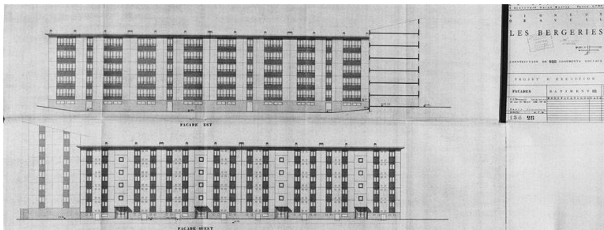
Bâtiment 18 (R + 5) : plans des façades est et ouest, dressés par J. L'Hernault, 30 janvier 1966. (AM Vigneux-sur-Seine, 80 W 29, dossiers 57-58)
