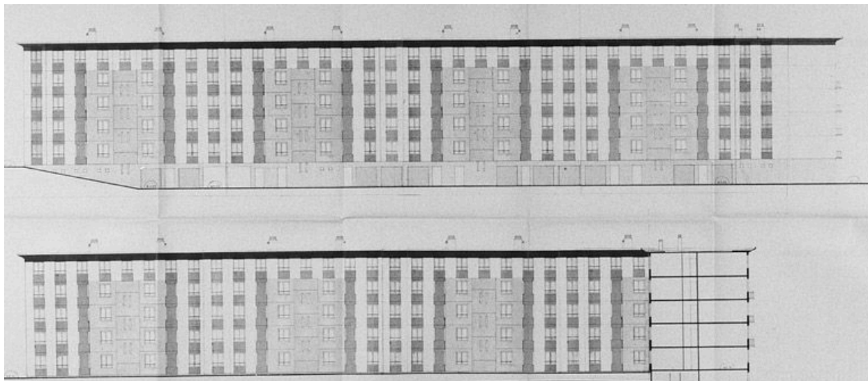
Bâtiment long R + 5 : plans des façades principales, dressés par J. L'Hernault, 16 juillet 1965. (AM Vigneux-sur-Seine, 80 W 29, dossiers 57-58)
