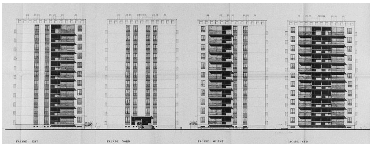
Bâtiments F, M et R (R + 10) : plans des quatre façades, dressés par J. L'Hernault, 16 juillet 1965. (AM Vigneux-sur-Seine, 80 W 29, dossiers 57-58)
