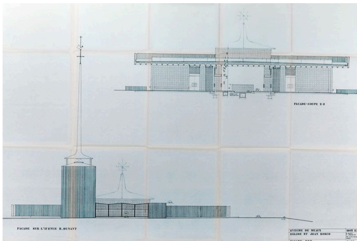
Projet de 1966. Coupe et élévation de la façade est. Plan ancien, 1 août 1966. (A Evêché Meaux)
