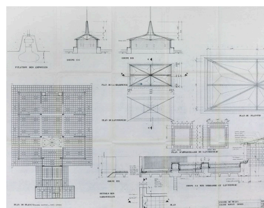
Projet de 1966. Coupes et plans de la dalle de couverture et du lanterneau. Plan ancien, 27 juillet 1966. (A Evêché Meaux) Autr. Michel (architecte) Marot IVR11_20117701143NUC4A
