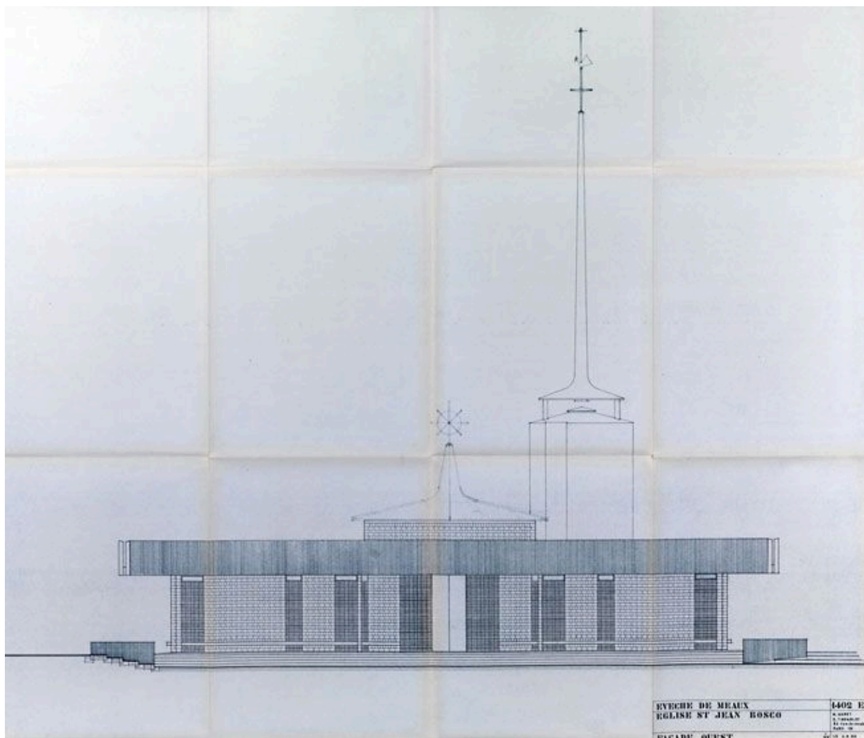
Projet de 1966. Elévation ouest (avec clocher-tour), 1/50. Plan ancien, 2 août 1966. (A Evêché Meaux)
