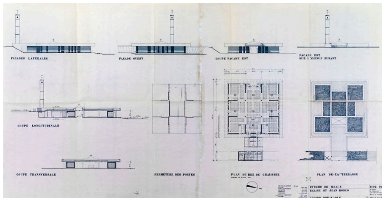
Projet de 1964. Plans de l'accord préalable au permis de construire, 1/200. Plan ancien, 20 novembre 1964. (A Evêché Meaux)
