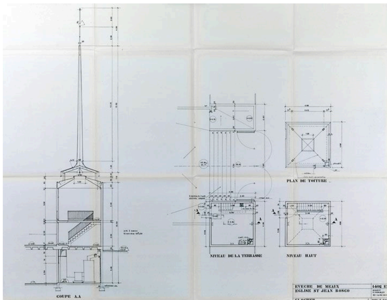
Projet de 1966. Coupe et plans de niveaux du clocher-tour, 1/50. Plan ancien, 10 août 1966. (A Evêché Meaux)
