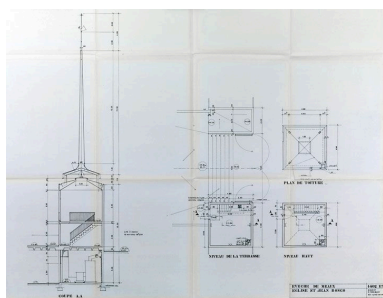
Projet de 1966. Coupe et plans de niveaux du clocher-tour, 1/50. Plan ancien, 10 août 1966. (A Evêché Meaux) Autr. Michel (architecte) Marot IVR11_20117701141NUC4A
