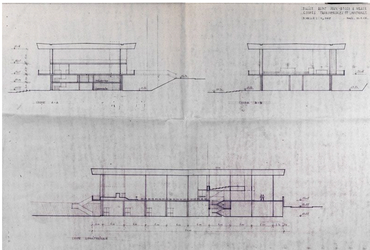
Avant-projet de forme rectangulaire. Coupes transversales et longitudinale. Plan ancien, 10 septembre 1963. (A Evêché Meaux)
