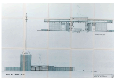
Projet de 1966. Coupe et élévation de la façade est. Plan ancien, 1 août 1966. (A Evêché Meaux) Autr. Michel (architecte) Marot IVR11_20117701142NUC4A
