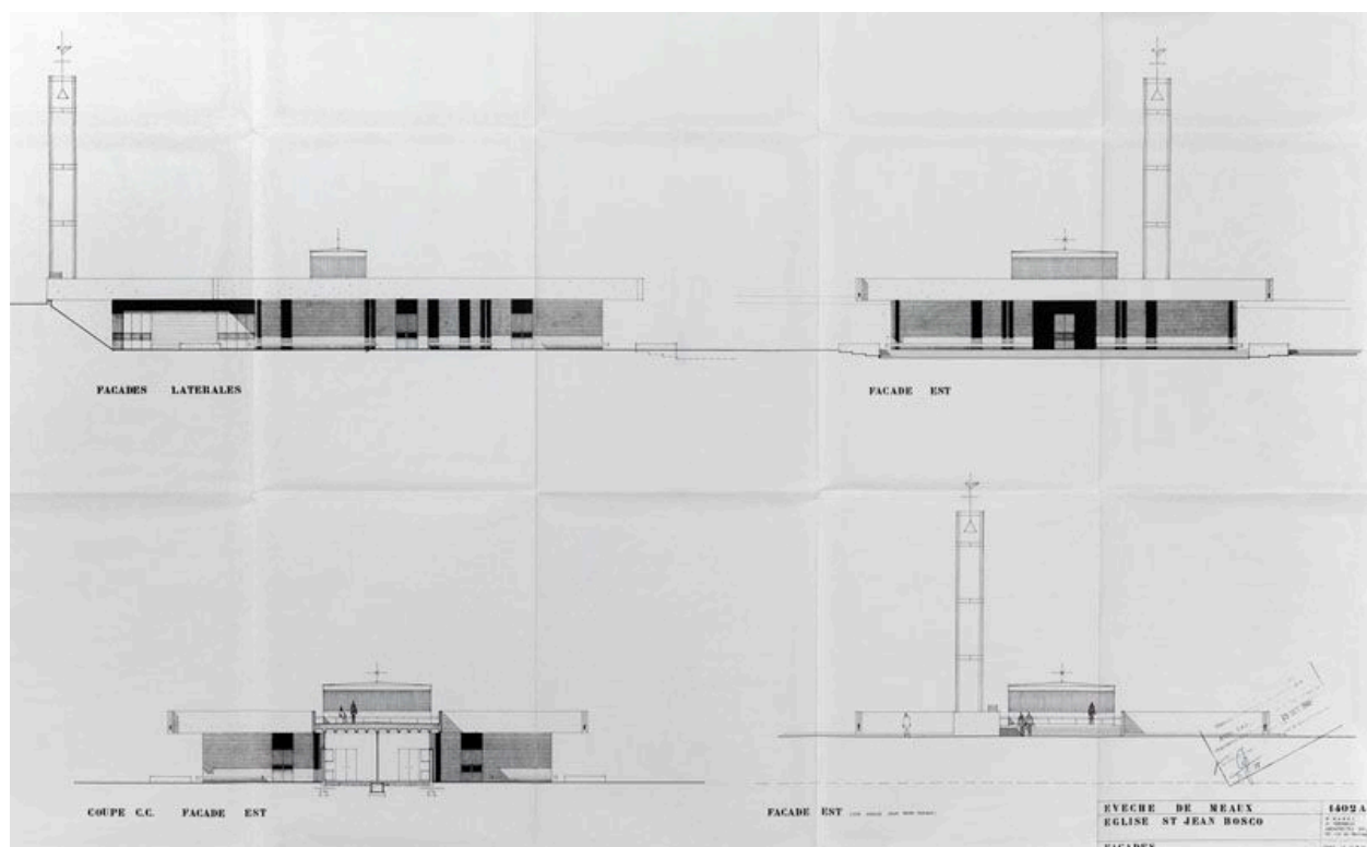
Projet de 1965. Elévations (avec haut-clocher), 1/100. Plan ancien, 14 août 1965. (A Evêché Meaux)
