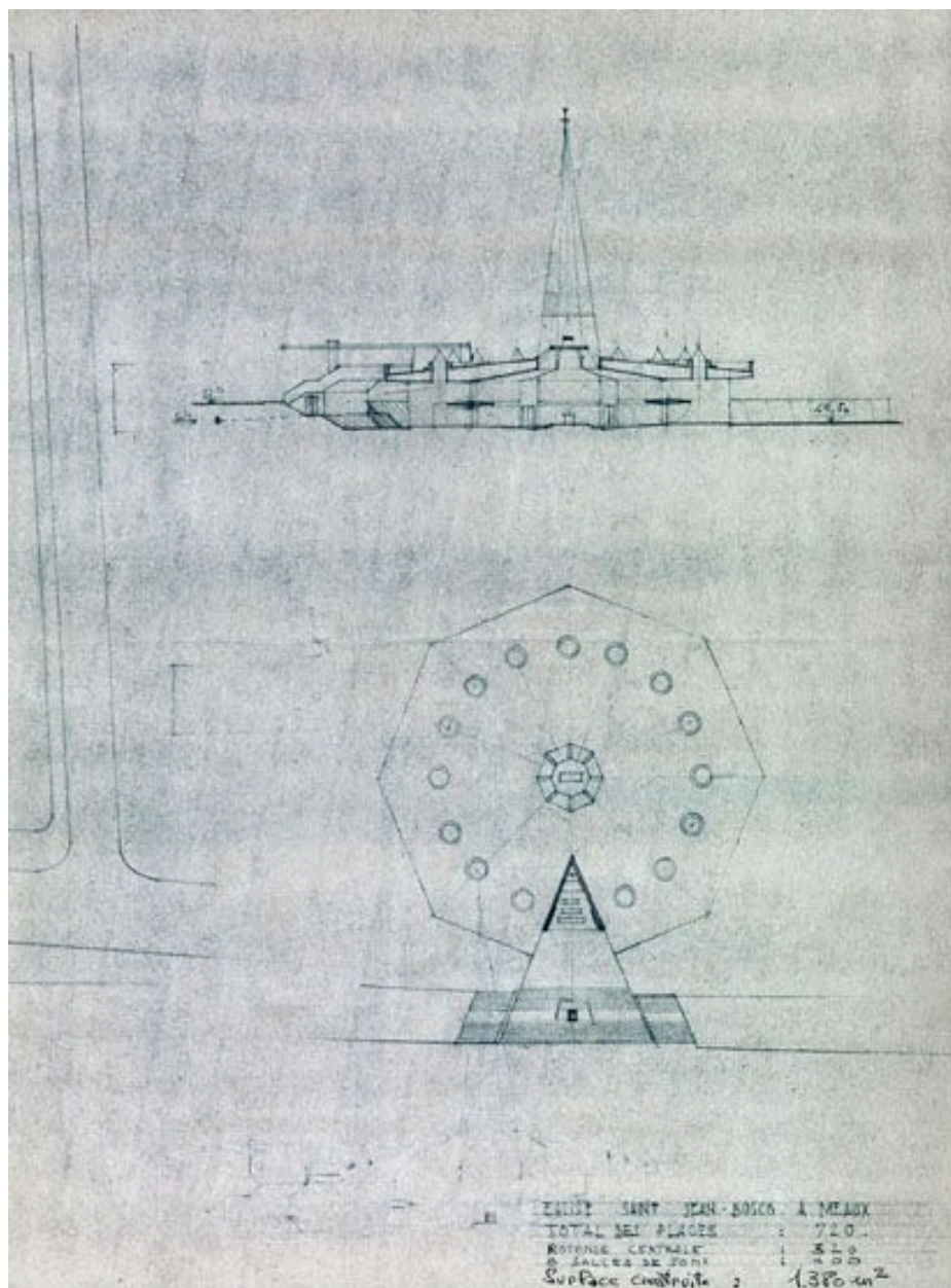
Avant-projet de forme octogonale. Coupe et plan de masse. Plan ancien, 1963. (A Evêché Meaux)
