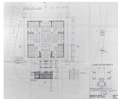
Projet de 1965. Plan du rez-de-chaussée, 1/100. Plan ancien, 14 août 1965. (A Evêché Meaux) Autr. Michel (architecte) Marot IVR11_20117701137NUC4A
