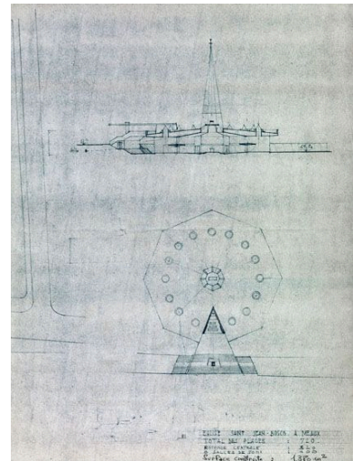
Avant-projet de forme octogonale. Coupe et plan de masse. Plan ancien, 1963. (A Evêché Meaux) Autr. Michel (architecte) Marot IVR11_20117701134NUC4A
