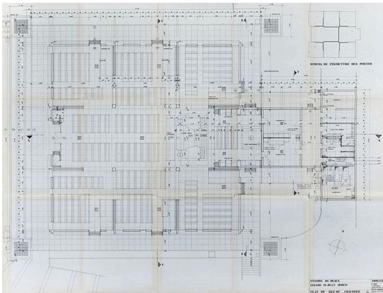
Projet de 1966. Plan du rez-de-chaussée, 1/50. Plan ancien, 13 juillet 1966. (A Evêché Meaux)
