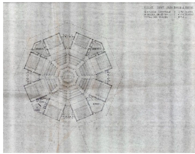
Avant-projet de forme octogonale. Plan de niveau. Plan ancien, 1963. (A Evêché Meaux) Autr. Michel (architecte) Marot IVR11_20117701132NUC4A
