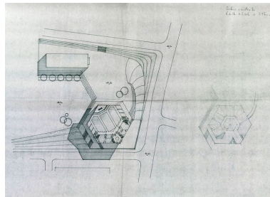
Avant-projet de forme hexagonale. Plan de masse. Plan ancien, 1963. (A Evêché Meaux) Autr. Michel (architecte) Marot IVR11_20117701133NUC4A
