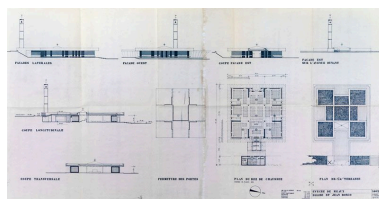
Projet de 1964. Plans de l'accord préalable au permis de construire, 1/200. Plan ancien, 20 novembre 1964. (A Evêché Meaux) Autr. Michel (architecte) Marot IVR11_20117701139NUC4A
