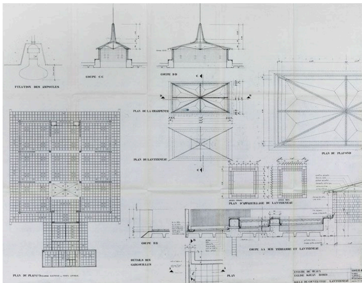
Projet de 1966. Coupes et plans de la dalle de couverture et du lanterneau. Plan ancien, 27 juillet 1966. (A Evêché Meaux)
