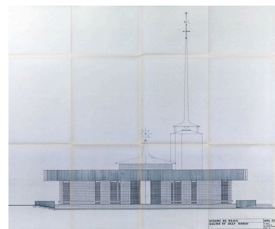
Projet de 1966. Elévation ouest (avec clocher-tour), 1/50. Plan ancien, 2 août 1966. (A Evêché Meaux) Autr. Michel (architecte) Marot IVR11_20117701140NUC4A
