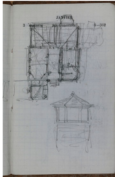
Projet de plan de la maison et de l'élévation du belvédère. Esquisse au crayon sur carnet, 3 janvier 1883. (Collection particulière de la famille Friesé, Carnets de P.E Friesé) Phot. Jean-Bernard Vialles, Autr. Paul (architecte) Friesé IVR11_20089500628NUC4A
