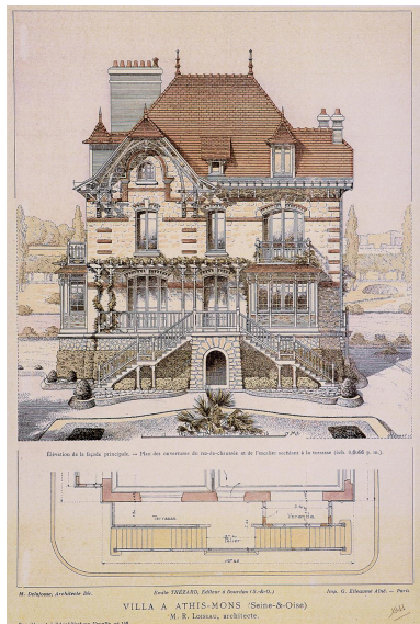
Elévation de la façade principale et plan des ouvertures du rez-de-chaussée et de l'escalier accédant à la terrasse, publiés dans "L'Architecture Usuelle", 1911, planche 148. IVR11_20029101139XA
