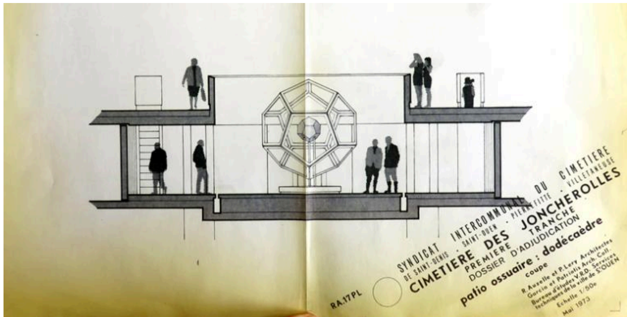
Coupe du patio de l'ossuaire et élévation du Dodécaèdre, dossier d'adjudication, mai 1973. SIAF/CAPA. Fonds Robert Auzelle 242 IFA, boîte 51, affaire RA 17.
