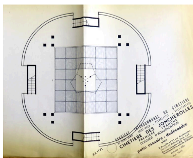
Plan du patio de l'ossuaire et emplacement du Dodécaèdre, dossier d'adjudication, mai 1973. SIAF/CAPA. Fonds Robert Auzelle 242 IFA, boîte 51, affaire RA 17. Phot. Isabelle Duhau, Autr. Robert (architecte) Auzelle IVR11_20179300261NUCA
