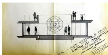
Coupe du patio de l'ossuaire et élévation du Dodécaèdre, dossier d'adjudication, mai 1973. SIAF/CAPA. Fonds Robert Auzelle 242 IFA, boîte 51, affaire RA 17. Phot. Isabelle Duhau, Autr. Robert (architecte) Auzelle IVR11_20179300262NUCA
