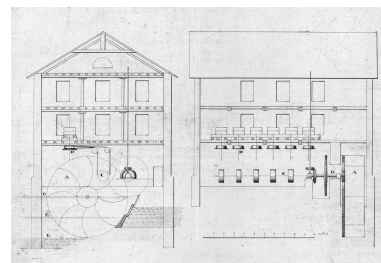
Coupes transversale et longitudinale montrant les mécanismes de transmission de l'énergie, s.d. [en note : projet 8 juil. 1854].
