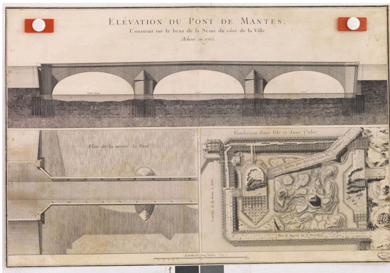
Elévation du pont de Mantes, construit sur le bras de la Seine du côté de la ville, achevé en 1765. Dessin, 3e quart 18e siècle. (AN, F/14 10206 3 dossier 8). On voit les trois arches caractéristiques du Pont Perronet du côté de Mantes, achevé en 1765.
