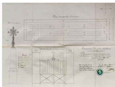
Plan général du cimetière avec le détail de la croix de cimetière et du portail d'entrée. Dessin, 1853. (AD Val d'Oise, 20Fi 59/10) Phot. Jean-Bernard Vialles, Autr. Heudebert (architecte) IVR11_20099500372NUC4A
