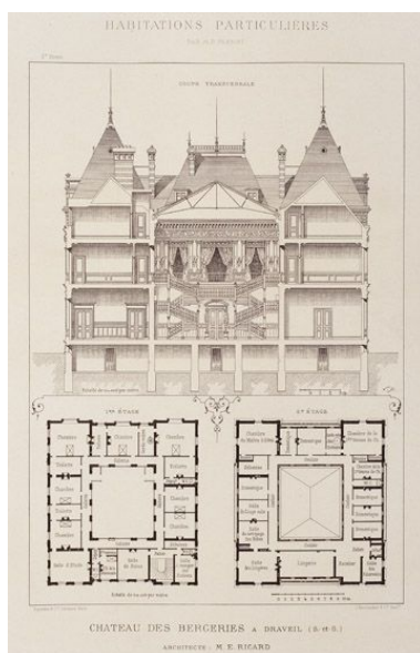
Coupe transversale et plans des 1er et 2e étages. Tiré de : Habitations particulières. Deuxième série. Maisons de campagne, villas et châteaux / P. Planat. Paris : Dujardin et Cie [ca 1890]. (BHVP, F° M° 32407) Autr. E. (architecte) Ricard IVR11_20069100202XA
