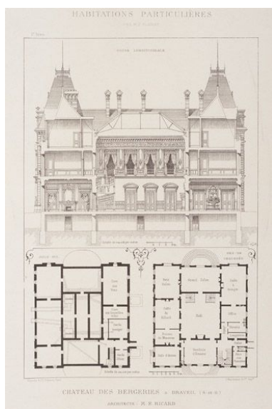
Coupe longitudinale et plans du sous-sol et du rez-de-chaussée. Tiré de : Habitations particulières. Deuxième série. Maisons de campagne, villas et châteaux / P. Planat. Paris : Dujardin et Cie [ca 1890]. (BHVP, F° M° 32407) Autr. E. (architecte) Ricard IVR11_20069100201XA
