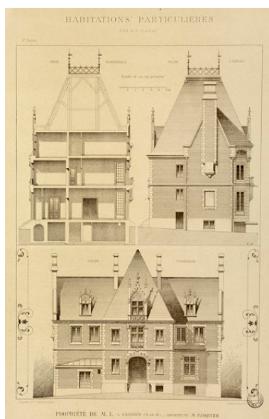
Elévation latérale droite, façade d'entrée dite sur le document "façade postérieure" et coupe transversale de la maison de "M.L.". Gravure. (AD Val d'Oise, 20Fi 59/15-17, en feuillet détaché)
