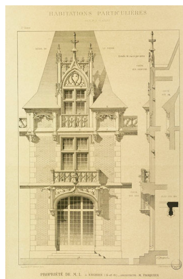
Elévation du pavillon central de la façade donnant sur le lac et coupes donnant le détail des différents éléments formant ressaut sur cette façade. Dessin. (AD Val d'Oise, 20Fi 59/15-17, en feuillet détaché)
