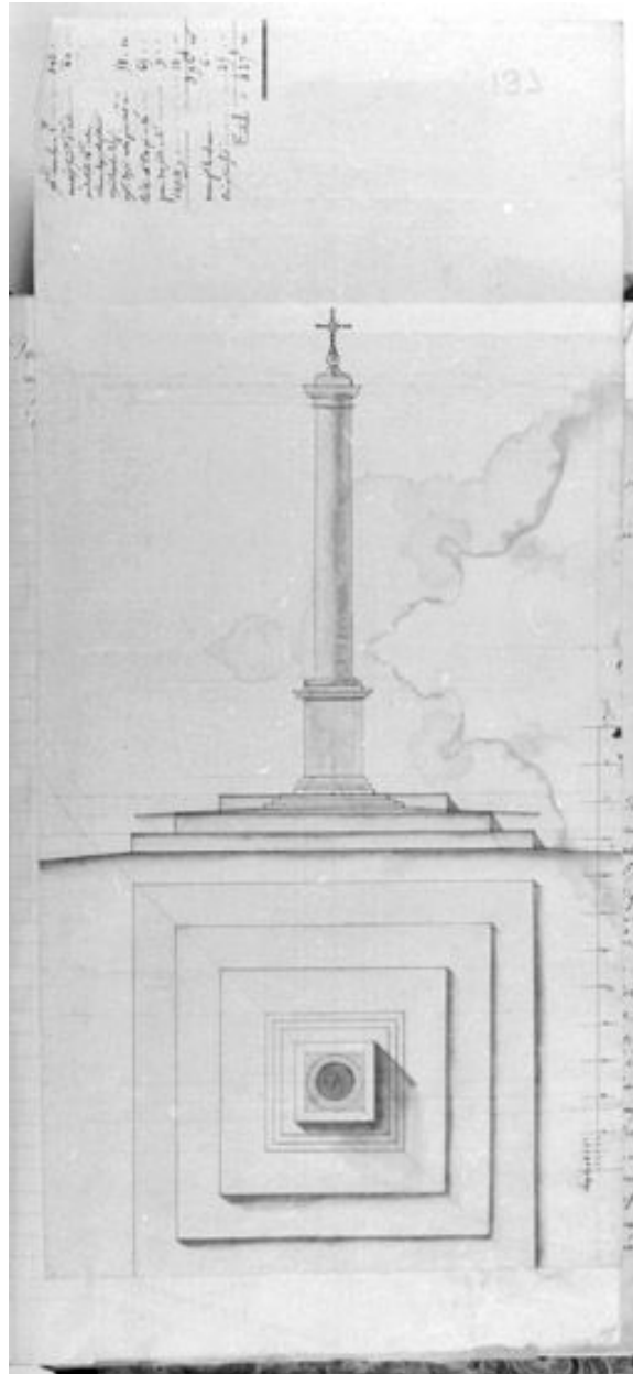
Projet de croix monumentale. AM de Mantes-la-Jolie. 2 S1.
