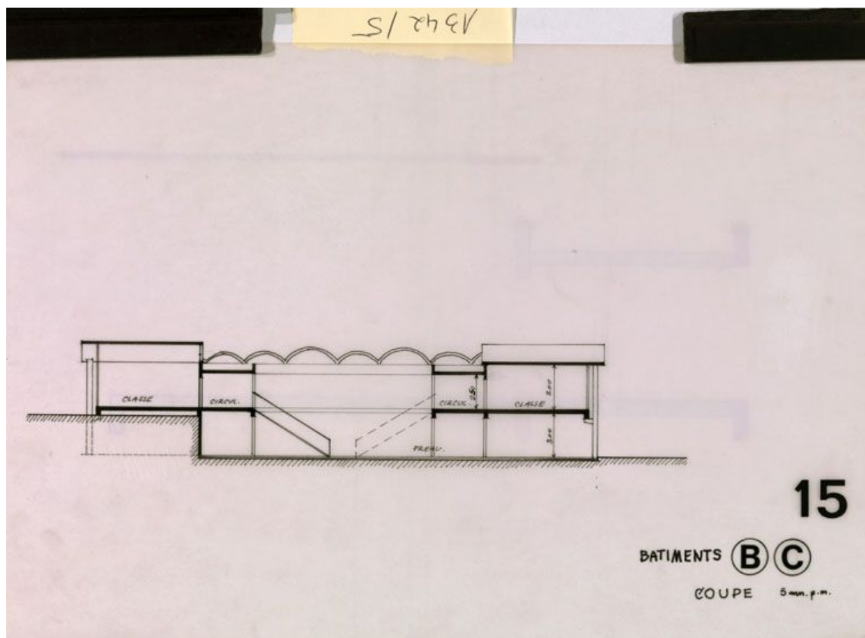
Groupe scolaire G3. coupe sur les bâtiments B et C du dossier d'avant-projet, 1972. Emile Aillaud, architecte. (Cité de l'architecture et du patrimoine, Archives d'architecture du XXe siècle).
