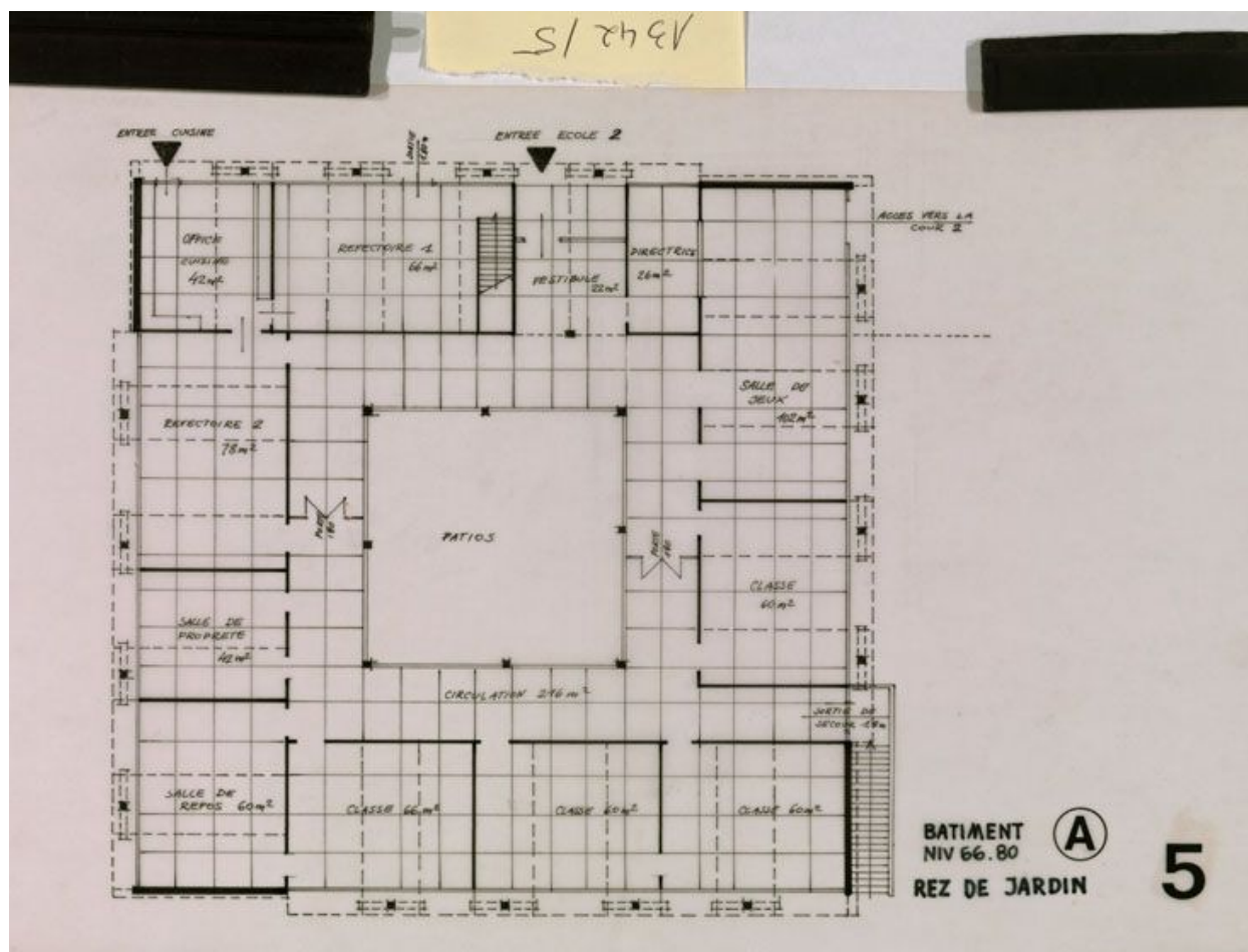
Groupe scolaire G3. Plan du rez de jardin du bâtiment A (école maternelle) du dossier d'avant-projet, 1972. Emile Aillaud, architecte. (Cité de l'architecture et du patrimoine, Archives d'architecture du XXe siècle).
