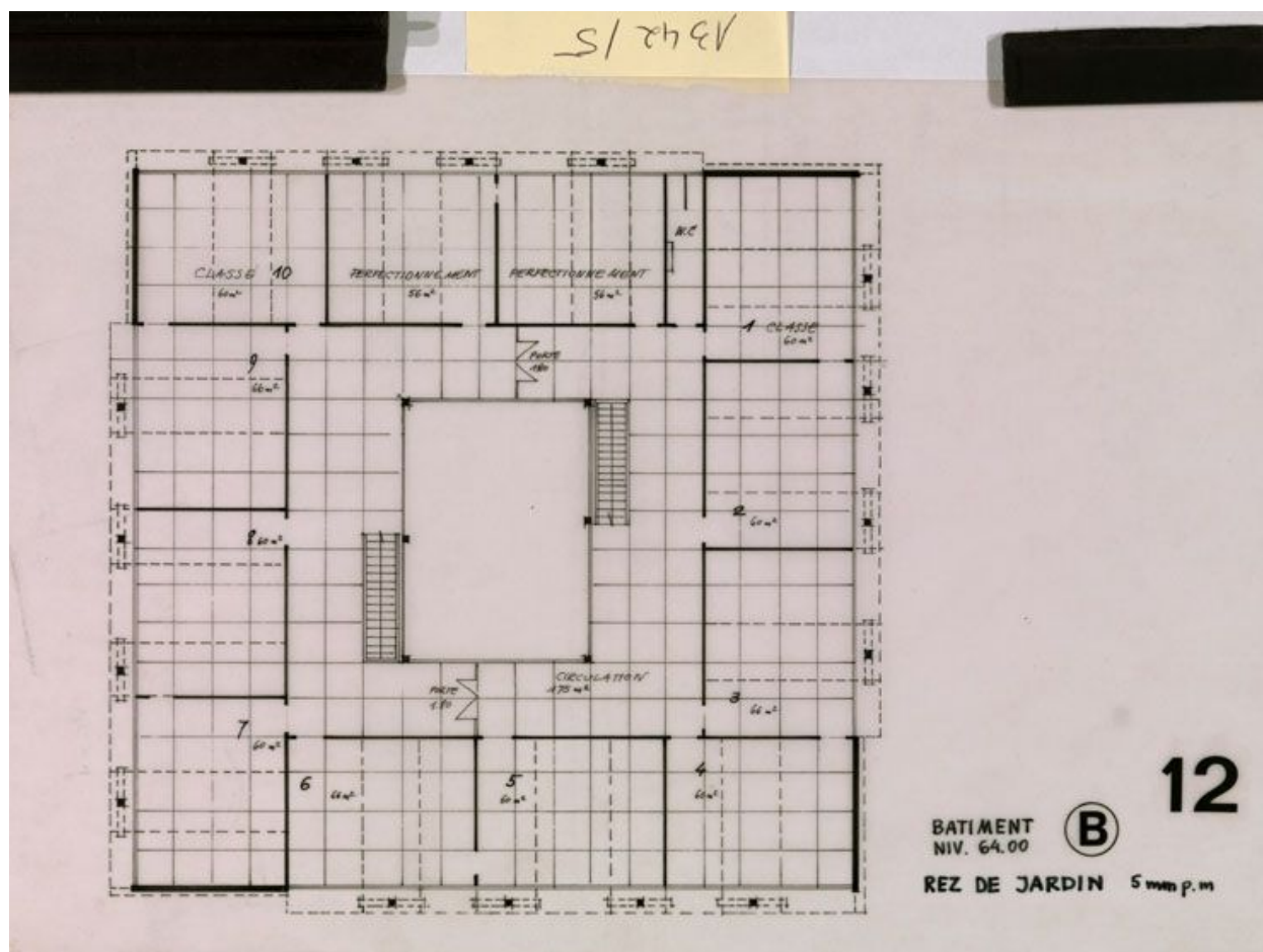
Groupe scolaire G3. Plan du rez de jardin du bâtiment B (école primaire) du dossier d'avant-projet, 1972. Emile Aillaud, architecte. (Cité de l'architecture et du patrimoine, Archives d'architecture du XXe siècle).
