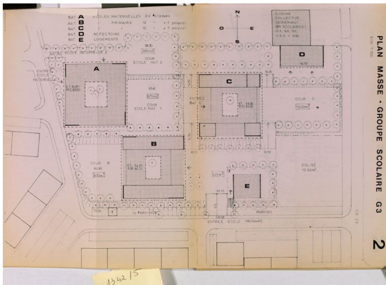
Groupe scolaire G3. Plan masse du dossier d'avant-projet, 1972. Emile Aillaud, architecte. (Cité de l'architecture et du patrimoine, Archives d'architecture du XXe siècle).
