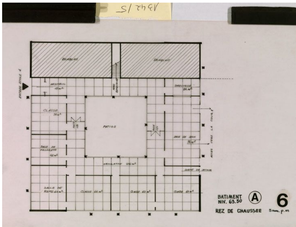
Groupe scolaire G3. Plan du rez de chaussée du bâtiment A (école maternelle) du dossier d'avant-projet, 1972. Emile Aillaud, architecte. (Cité de l'architecture et du patrimoine, Archives d'architecture du XXe siècle).
