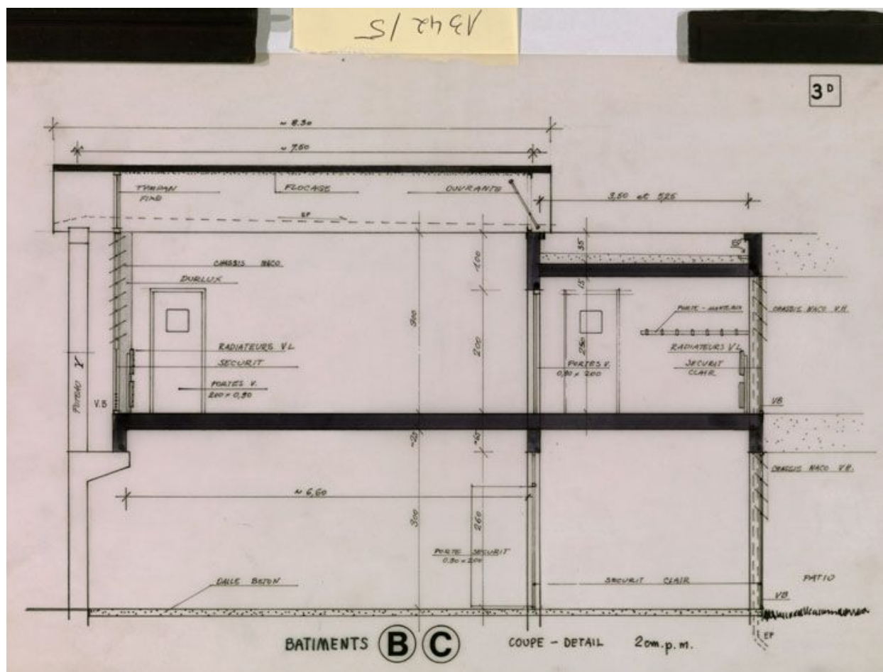
Groupe scolaire G3. Détail de coupe sur les bâtiments B et C du dossier d'avant-projet, 1972. Emile Aillaud, architecte. (Cité de l'architecture et du patrimoine, Archives d'architecture du XXe siècle).
