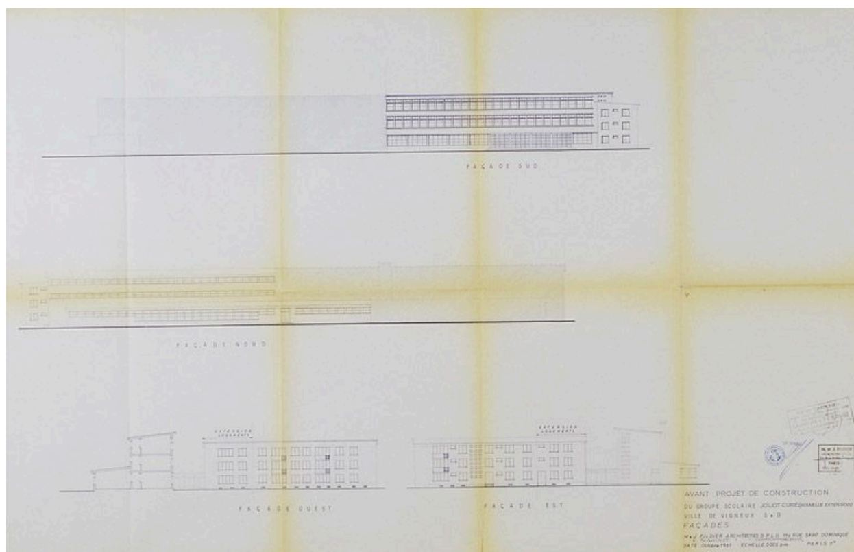
Avant-projet de construction de la nouvelle extension : façades sud et nord du bâtiment scolaire ; façades est et ouest du bâtiment de logements. (AM Vigneux-sur-Seine, 1 M 114)
